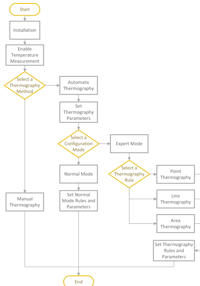
Abbildung 7-1 Flussdiagramm zur Konfiguration der Thermografie
