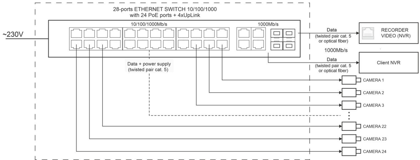
Abb. 1. Blockdiagramm.
