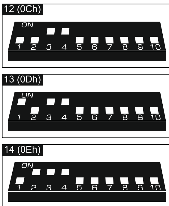
Abb. 6. Einstellung der DIP-Schalter im Modul INT-E.
