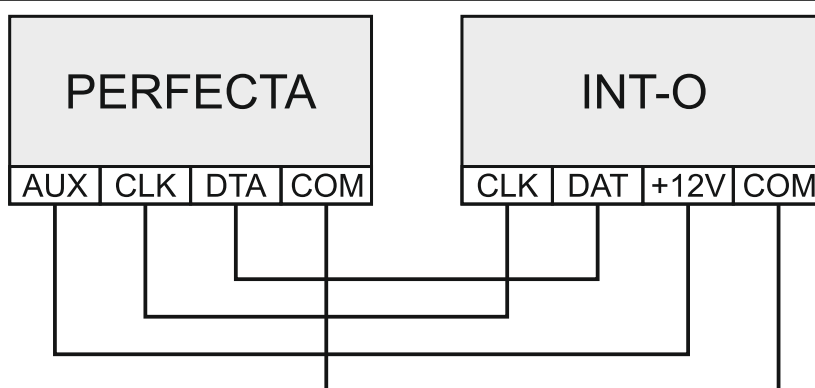
Abb. 7. Anschluss des Moduls INT-O an die Zentrale.
