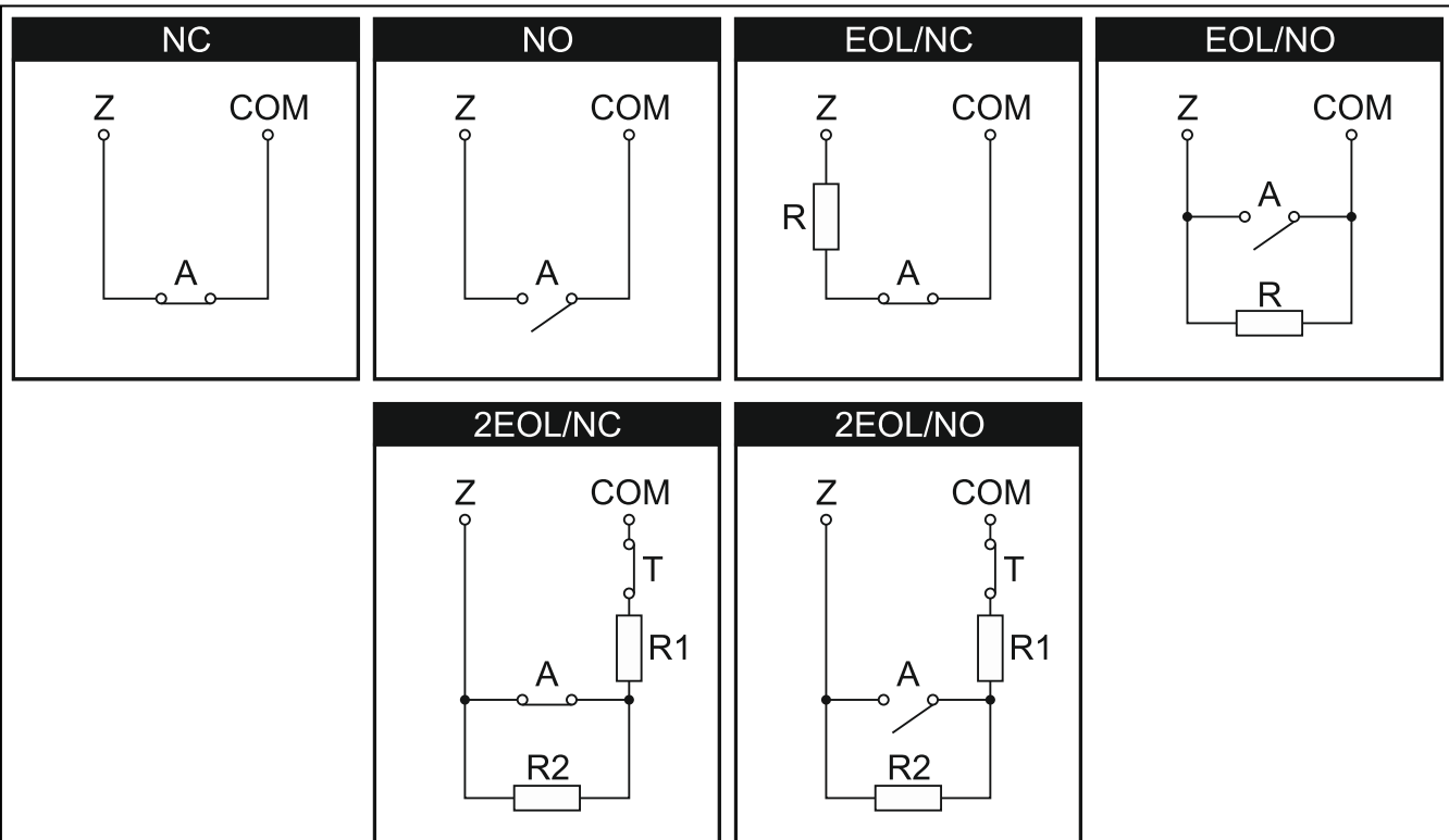
Abb. 9. Anschluss der Melder an die Meldelinien. Die Ausgänge des Melders sind mit folgenden Buchstaben gekennzeichnet: A – Alarm, T – Sabotage.
