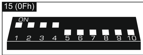
Abb. 8. Einstellung der DIP-Schalter im Modul INT-O.
