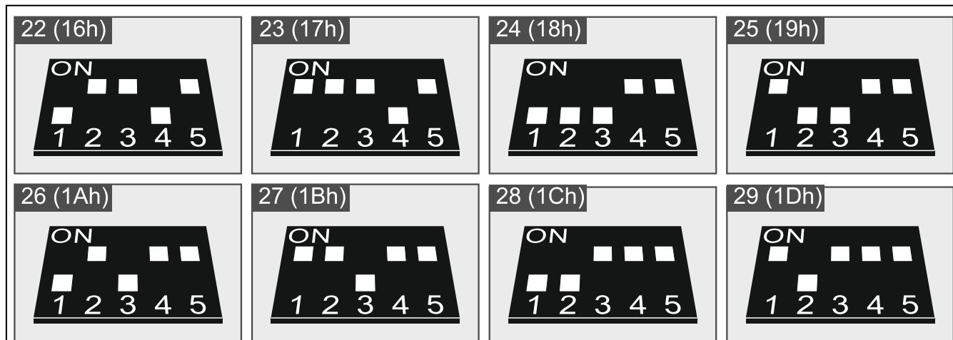
Abb. 20. Einstellung der DIP-Schalter im Modul INT-CR.
