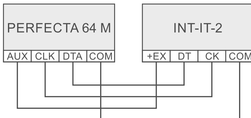
Abb. 18. Anschluss des Moduls INT-IT-2 an die Zentrale.
