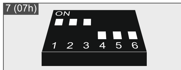
Abb. 12. Einstellung der DIP-Schalter im Erweiterungsmodul INT-RX-S.
