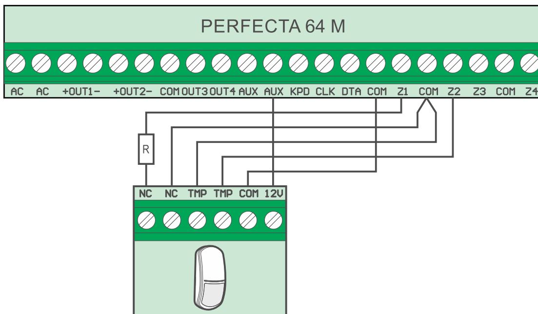
Abb. 23. Beispiel für den Anschluss eines NC-Melders in der Konfiguration EOL.
