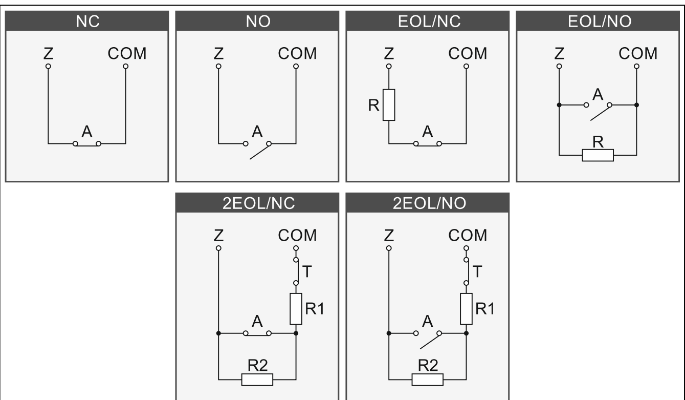
Abb. 21. Anschluss der Melder an die Meldelinien. Die Ausgänge des Melders sind mit folgenden Buchstaben gekennzeichnet: A – Alarm, T – Sabotage.
