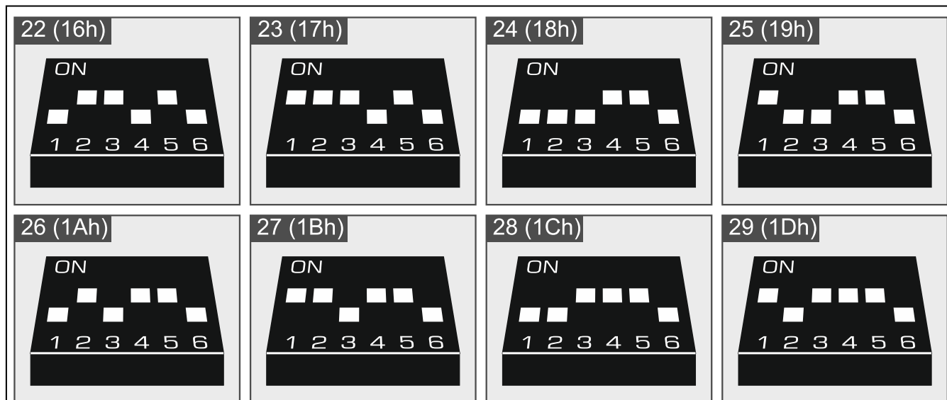
Abb. 19. Einstellung der DIP-Schalter im Modul INT-IT-2.
