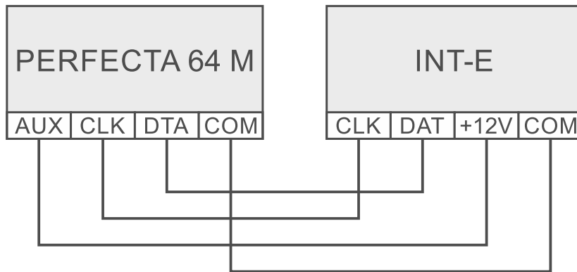
Abb. 13. Anschluss des Erweiterungsmoduls INT-E an die Zentrale.
