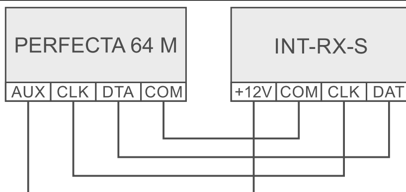
Abb. 11. Anschluss des Erweiterungsmoduls INT-RX-S an die Zentrale.
