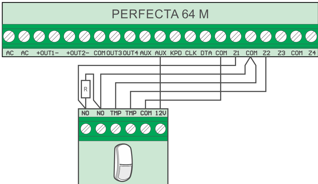
Abb. 24. Beispiel für den Anschluss eines NO-Melders in der Konfiguration EOL.
