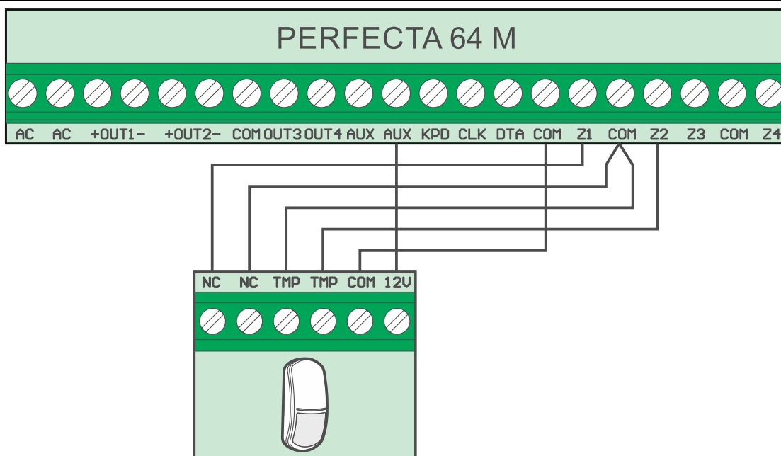
Abb. 22. Beispiel für den Anschluss eines NC-Melders (den NO-Melder schließen Sie identisch an).
