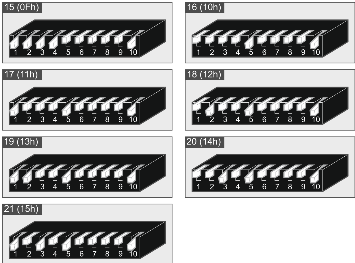
Abb. 17. Einstellung der DIP-Schalter im Erweiterungsmodul INT-ORS.
