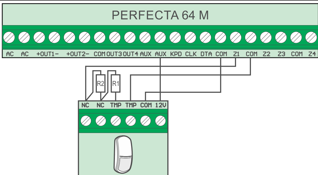
Abb. 25. Beispiel für den Anschluss eines NC-Melders in der Konfiguration 2EOL (den NO-Melder schließen Sie identisch an).
