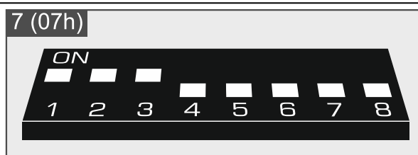
Abb. 8. Einstellung der DIP-Schalter im Modul INT-RX-S.
