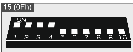
Abb. 12. Einstellung der DIP-Schalter im Modul INT-O.
