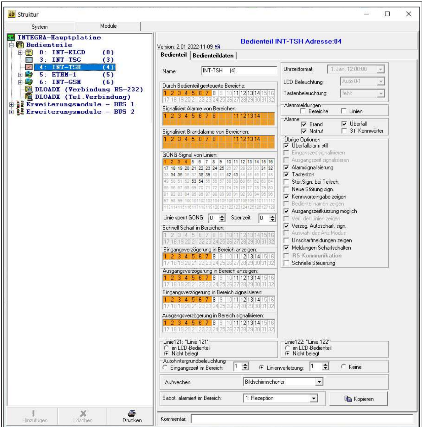
Abb. 26. Programm DLOADX: Bedienteil im INTEGRA System – Registerkarte „Bedienteil“ (Beispieleinstellungen).
