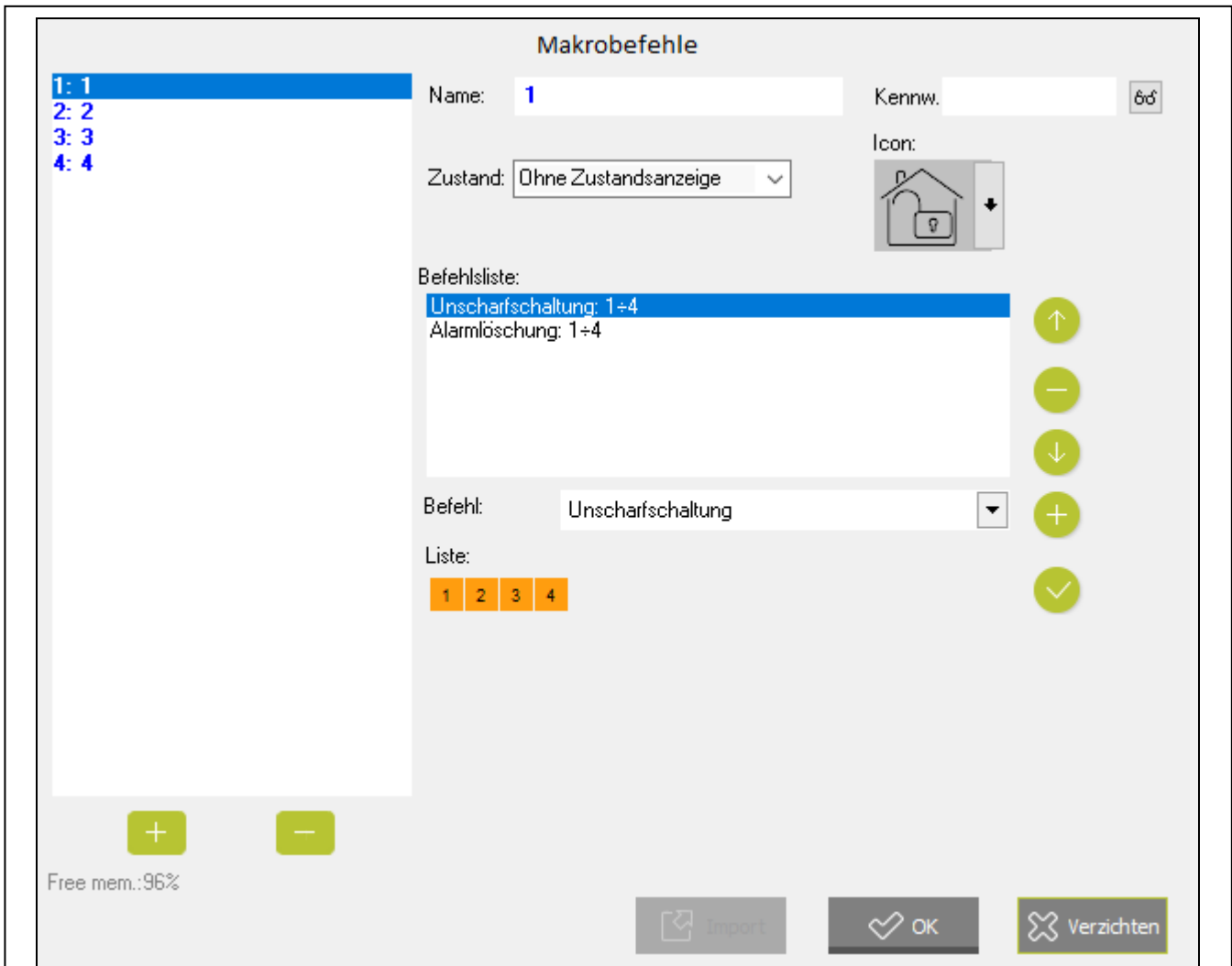
Abb. 40. Programm PERFECTA SOFT: Fenster „Makrobefehle“ (Werkseinstellungen).
