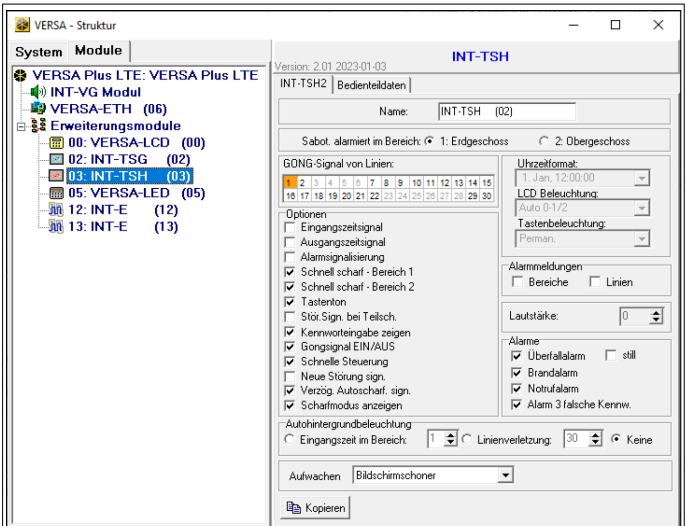
Abb. 44. Programm DLOADX: Bedienteil im VERSAs System – Registerkarte „INT-TSH2“ (Beispiel).
