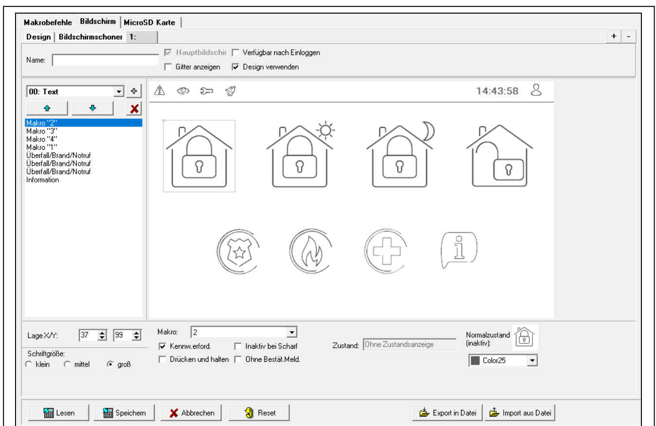
Abb. 30. Programm DLOADX: Registerkarte, die den Benutzerbildschirm präsentiert (Werkseinstellungen).
