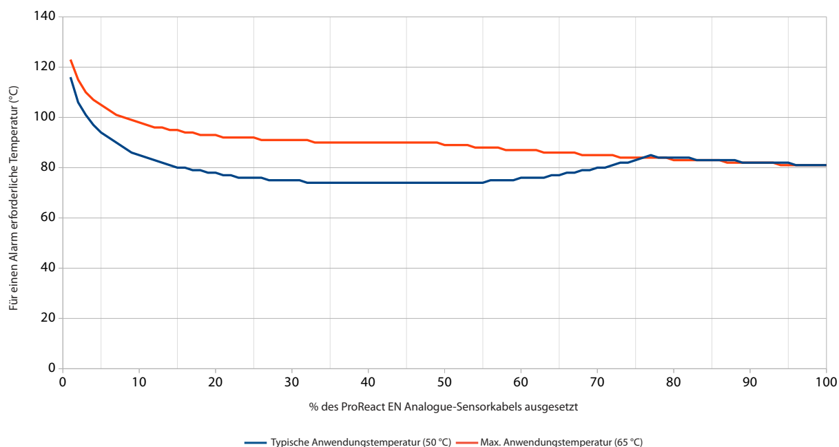
Diagramm A6 - Die für einen Alarm erforderliche erwartete Temperatur im Verhältnis zum prozentualen Anteil der 100°C-Einstellung des ProReact EN Analogue-LHD-Kabels
