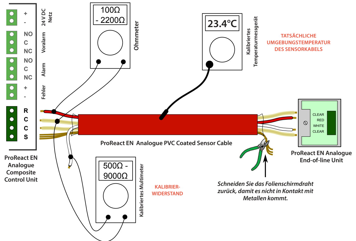
Abbildung 10: Typischer Systemschaltplan für das ProReact EN Analogue-LHD-System
