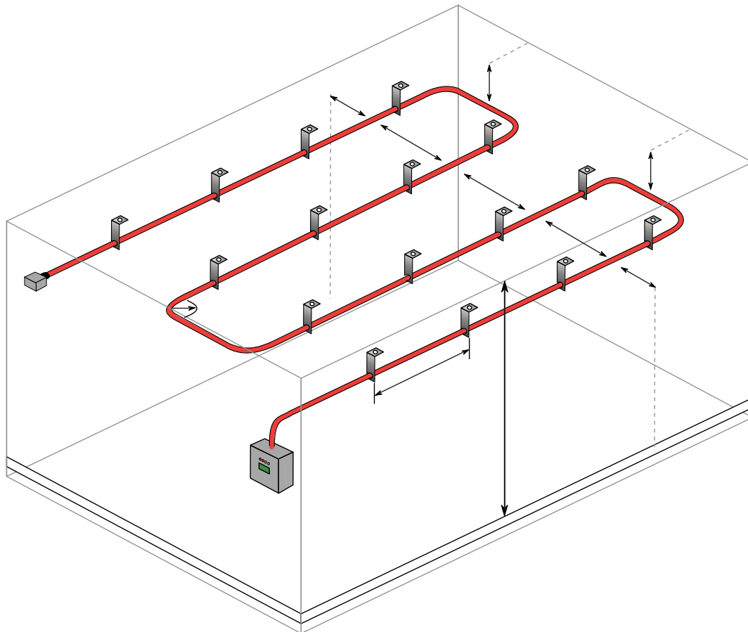
Abbildung 8: Raumschutz mit dem ProReact-EN Analogue-LHD-System
