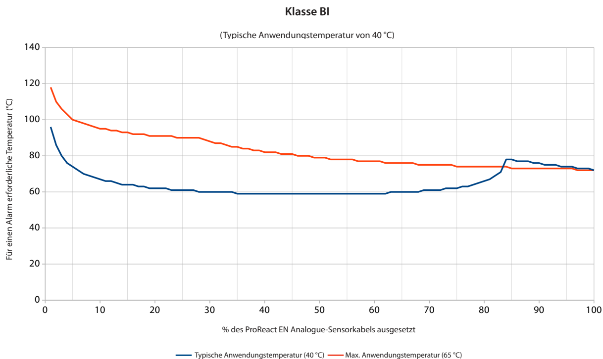
Diagramm 2 - Die für einen Alarm erforderliche erwartete Temperatur im Verhältnis zum prozentualen Anteil der Klasse-BI-Einstellung des ProReact EN Analogue-LHD-Kabels
