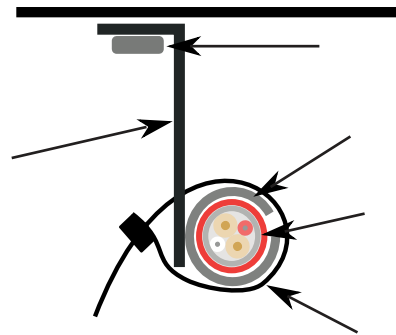
Abbildung 7: Empfohlene Befestigung des ProReact EN Analogue-Sensorkabels an einer Decke oder flachen Oberfläche
