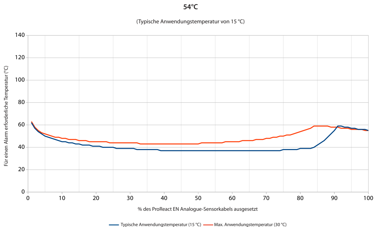
Diagramm A1 - Die für einen Alarm erforderliche erwartete Temperatur im Verhältnis zum prozentualen Anteil der 54°C-Einstellung des ProReact EN Analogue LHD-Kabels
