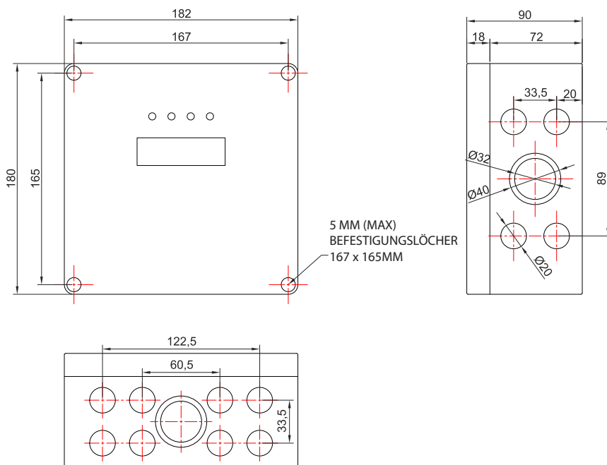
Abbildung 2. Maßzeichnung – ProReact EN Analogue Composite Control Unit
