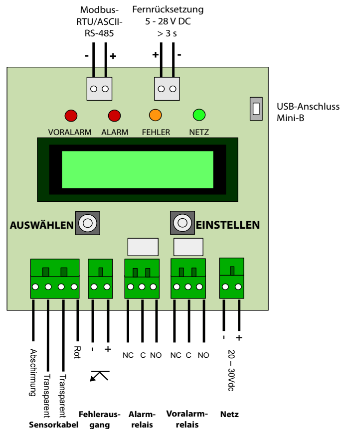
Abbildung 9: PCB-Schaltplan
