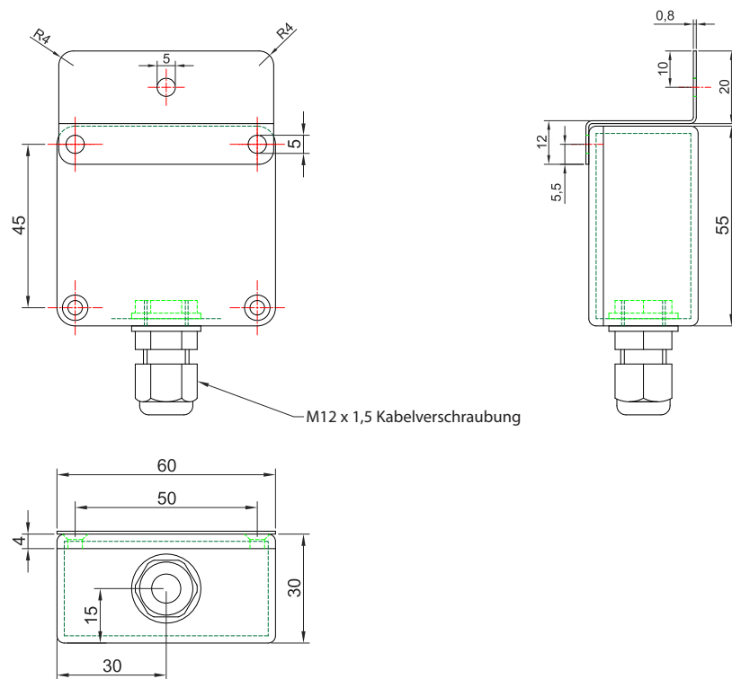
Abbildung 3. Maßzeichnung – ProReact EN Analogue End-of-line Unit
