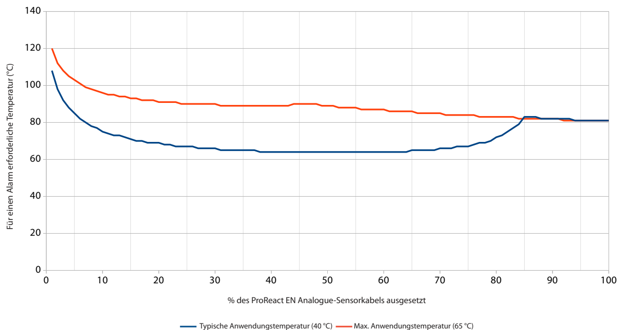
Diagramm A5 - Die für einen Alarm erforderliche erwartete Temperatur im Verhältnis zum prozentualen Anteil der 86°C-Einstellung des ProReact EN Analogue-LHD-Kabels
