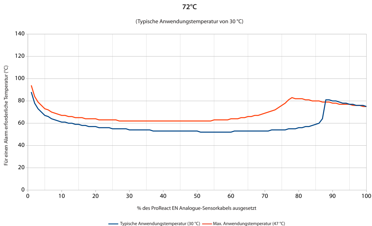
Diagramm A3 - Die für einen Alarm erforderliche erwartete Temperatur im Verhältnis zum prozentualen Anteil der 72°C-Einstellung des ProReact EN Analogue-LHD-Kabels
