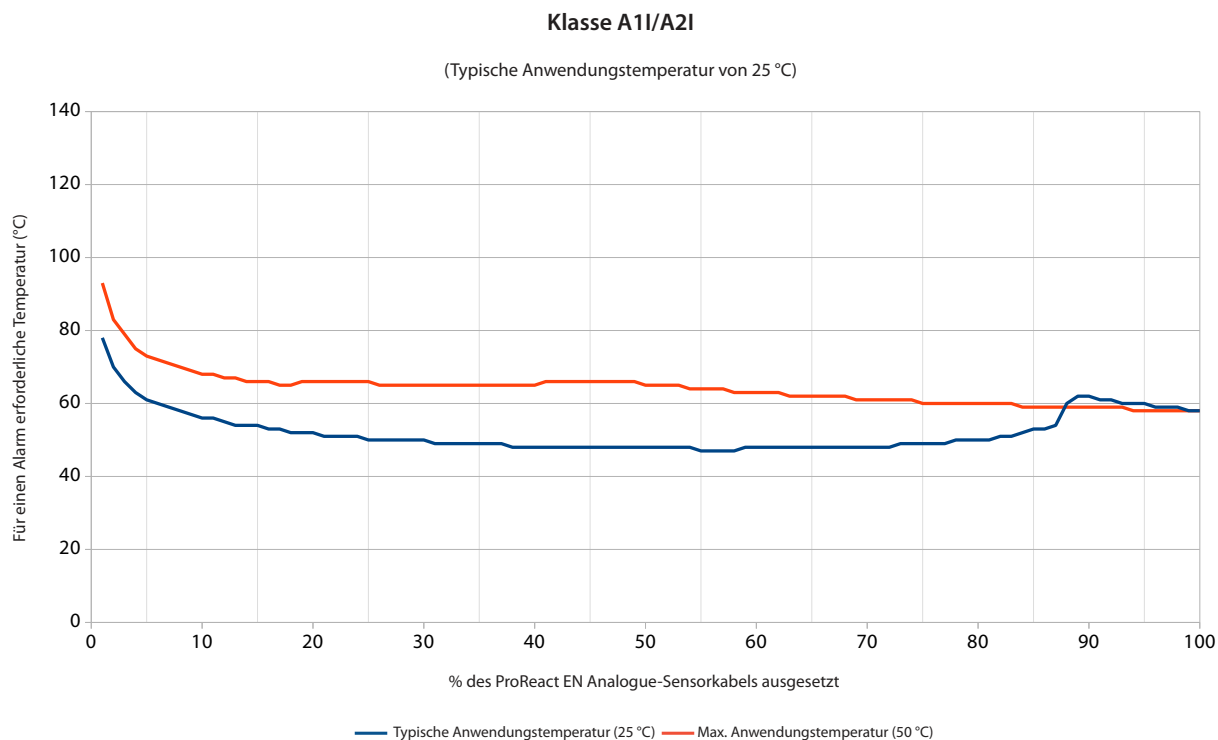
Diagramm 1 - Die für einen Alarm erforderliche erwartete Temperatur im Verhältnis zum prozentualen Anteil der Klasse-A1I/A2I-Einstellung des ProReact EN Analogue-LHD-Kabels
