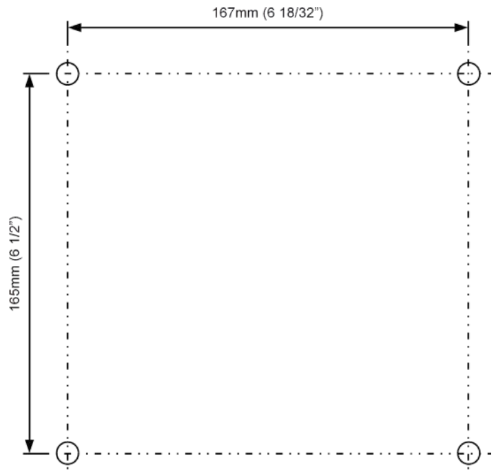
Abbildung 5: Befestigungsmaße für die Montage der ProReact EN Analogue Composite Control Unit
