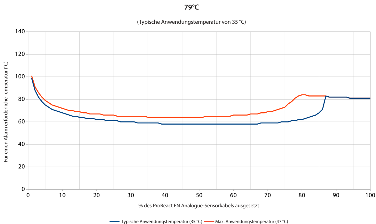
Diagramm A4 - Die für einen Alarm erforderliche erwartete Temperatur im Verhältnis zum prozentualen Anteil der 79°C-Einstellung des ProReact EN Analogue LHD-Kabels
