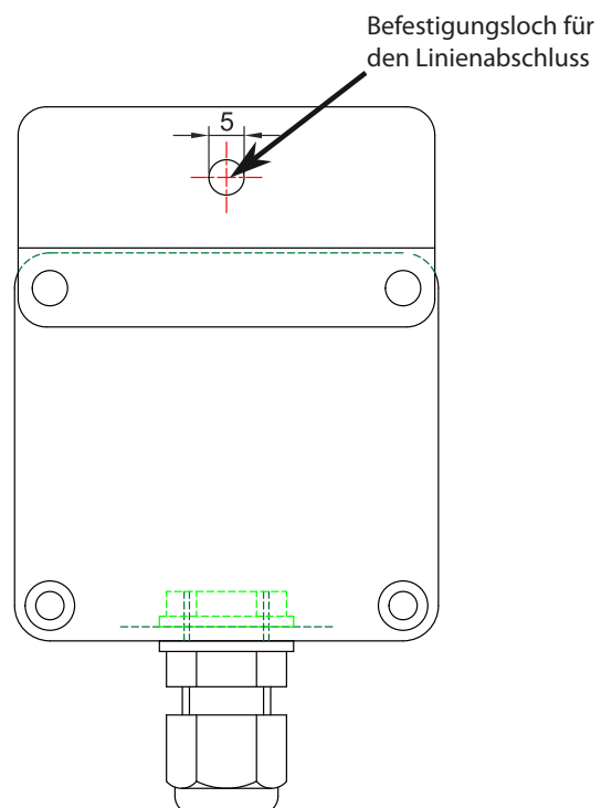
Abbildung 6: Befestigungsmaße für die Montage des ProReact EN Analogue End-of-line Unit
