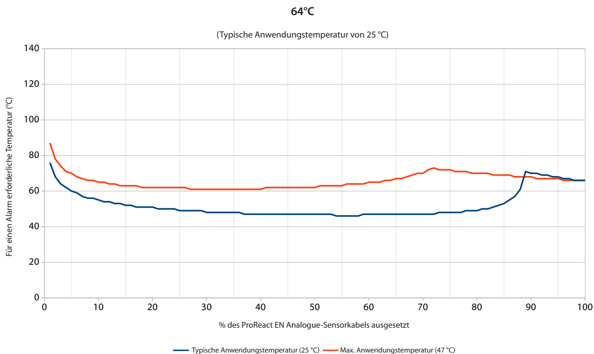
Diagramm A2 - Die für einen Alarm erforderliche erwartete Temperatur im Verhältnis zum prozentualen Anteil der 64°C-Einstellung des ProReact EN Analogue LHD-Kabels
