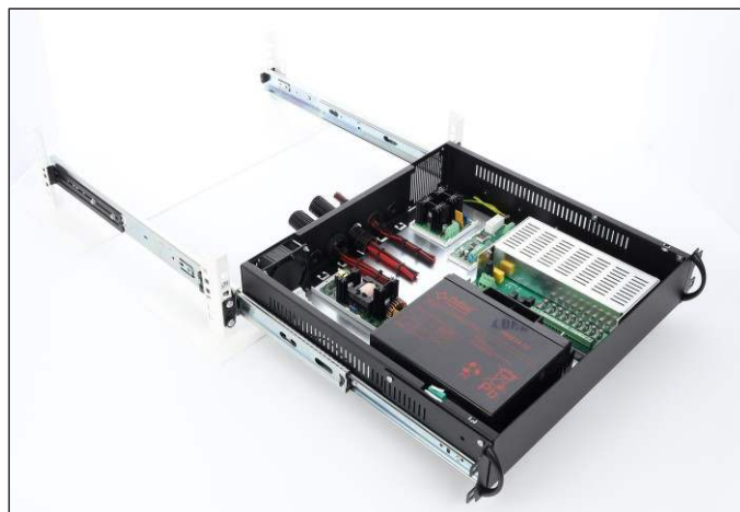
Gehäuse mit Schieber in die im 19"-RACK-Schrank installierten Schienen schieben
