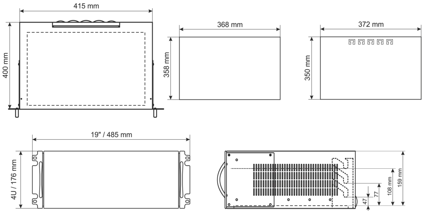
Abbildung 2. Abmessungen.
