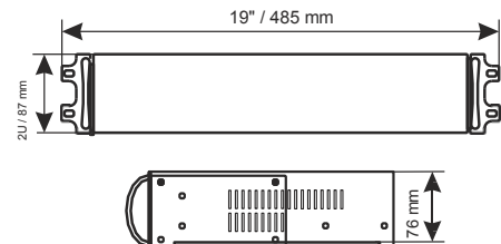
Montage auf einer ARAS600N/800N/1000N- Schiene
