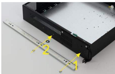
Befestigen Sie die Schieber mit zwei Schrauben am ARAD-Gehäuse (vergessen Sie nicht die Unterlegscheibe unter der zweiten Schraube)
