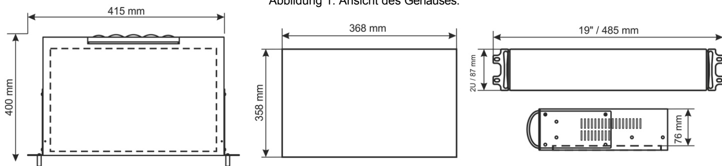
Abbildung 2. Abmessungen.
