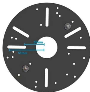
Bohrradius 30 - 51 mm
