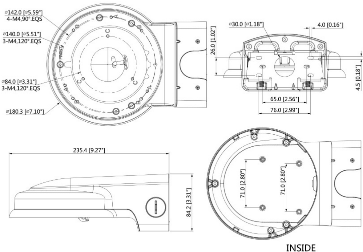
Abmessungen
