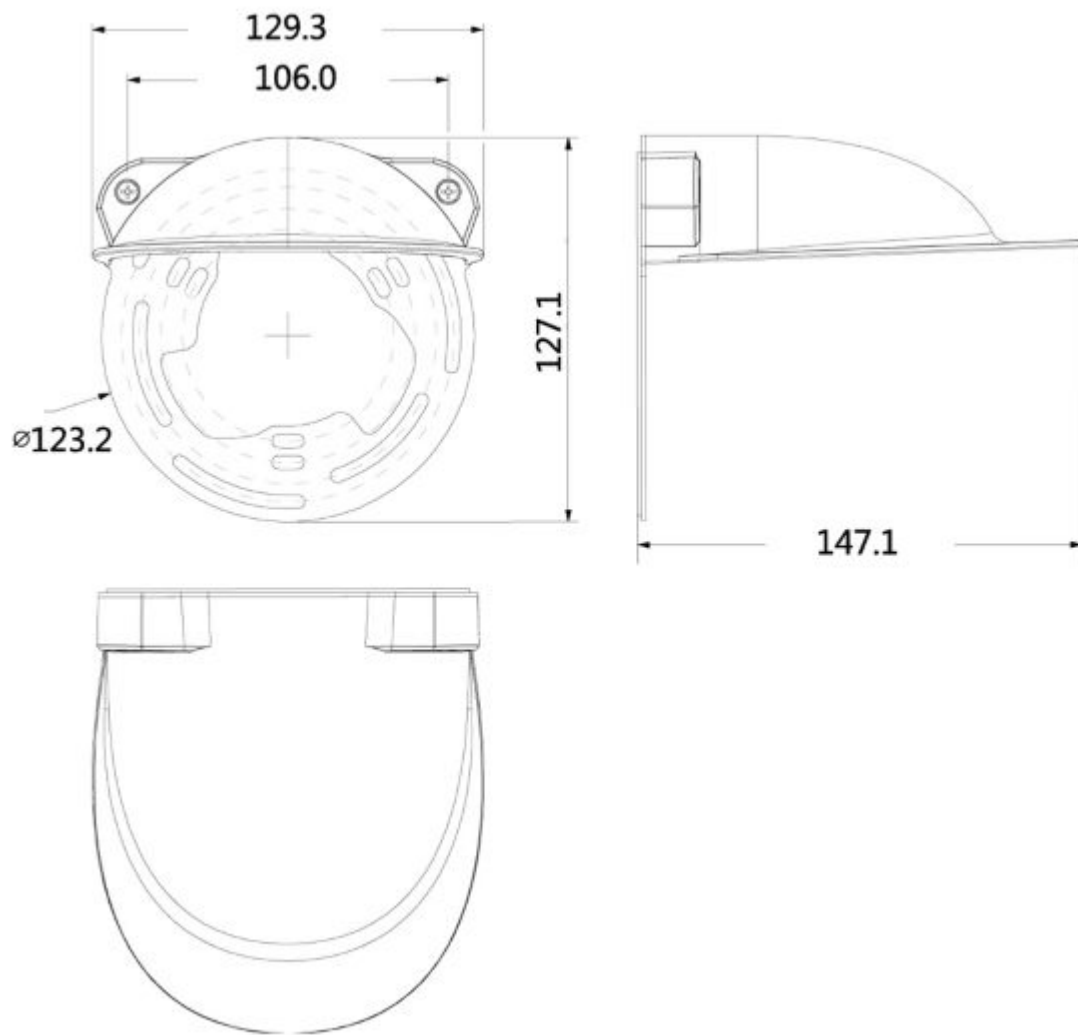
Abmessungen
