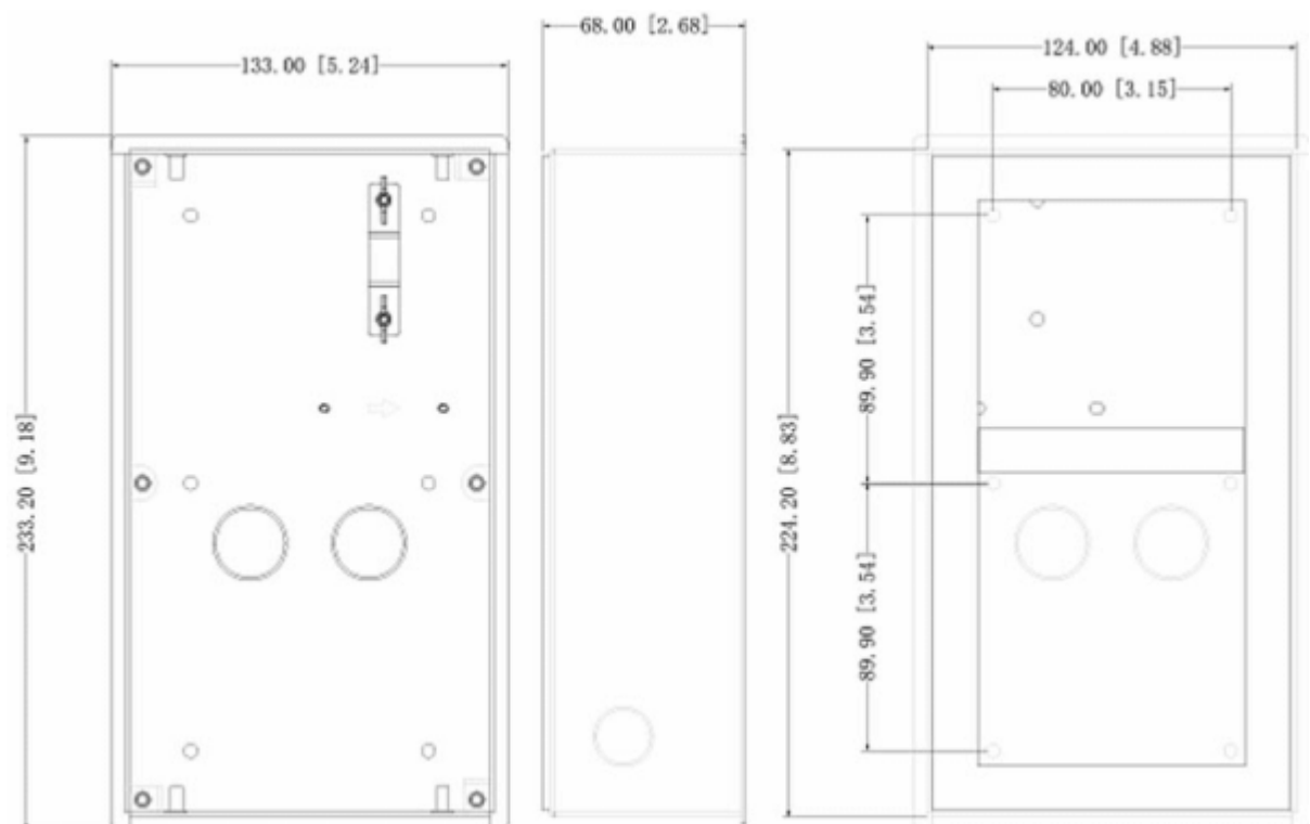
Abmessungen
