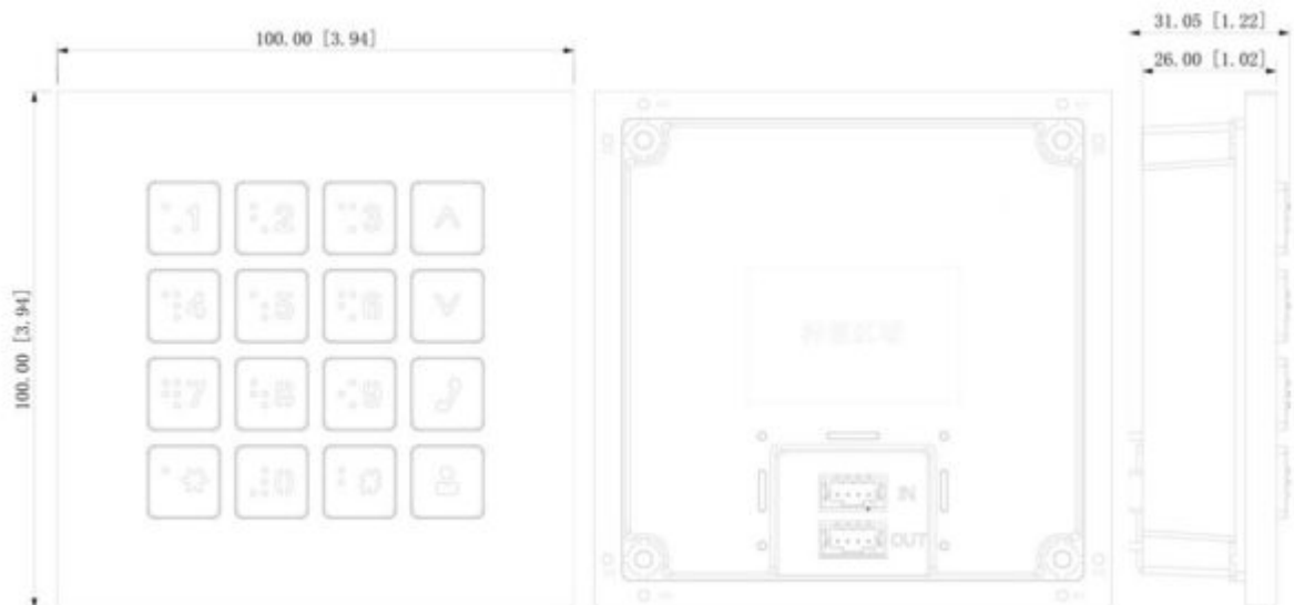
Abmessungen
