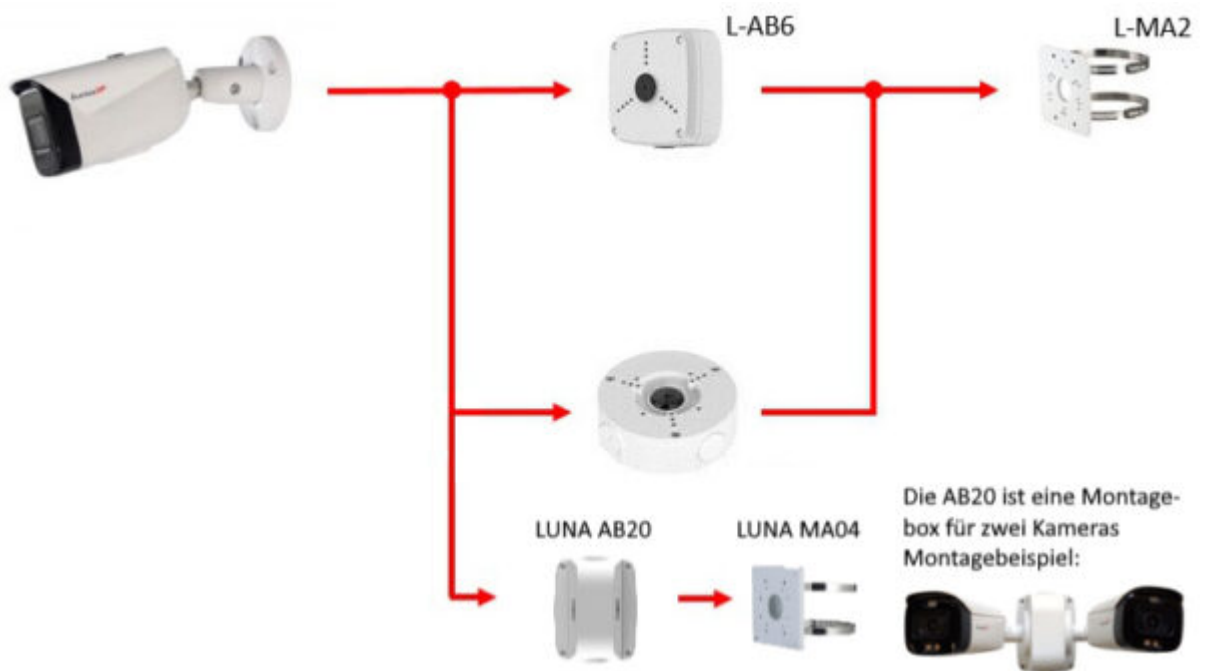
Montageoptionen
