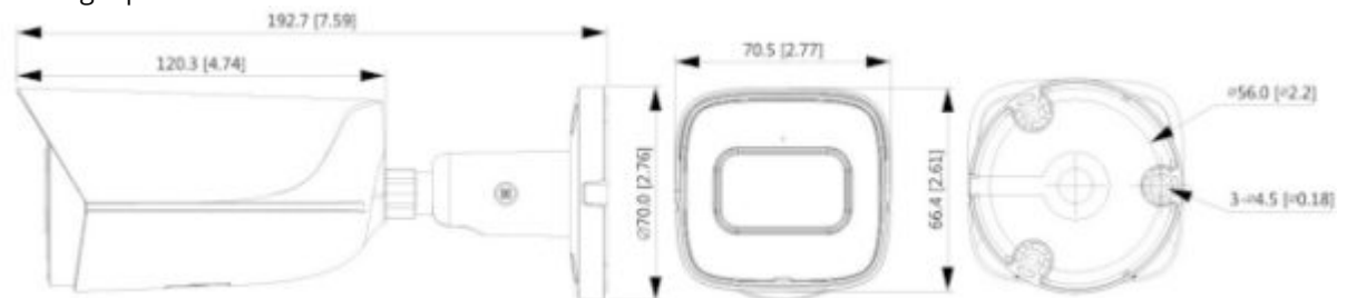
Abmessungen
