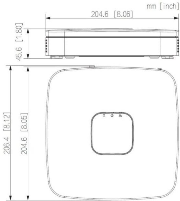
Abmessungen
