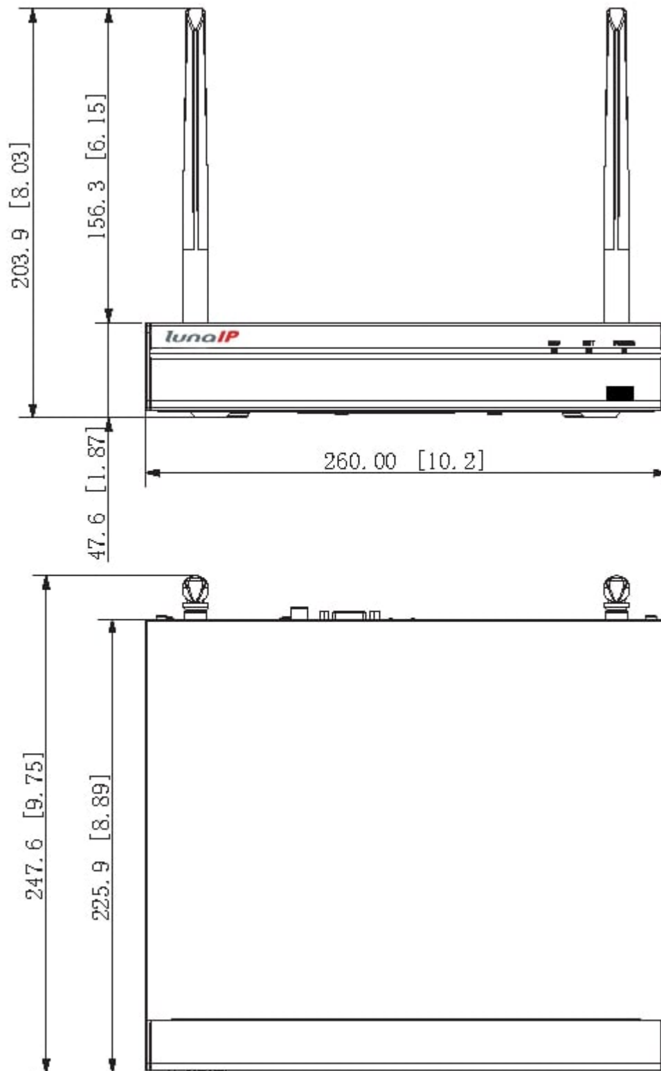
Abmessungen
