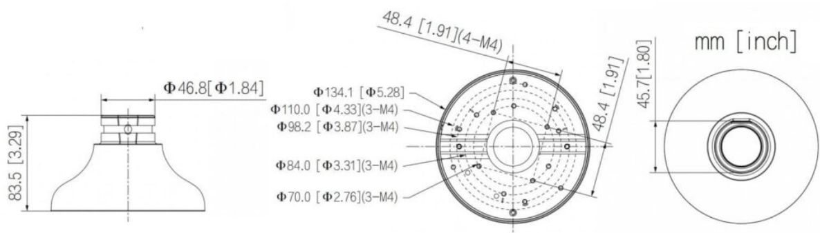
Abmessungen
