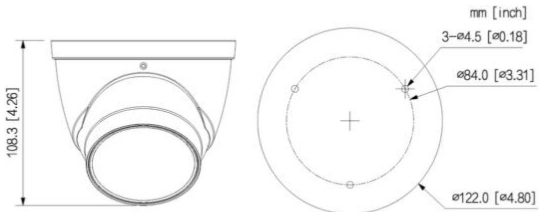
Abmessungen
