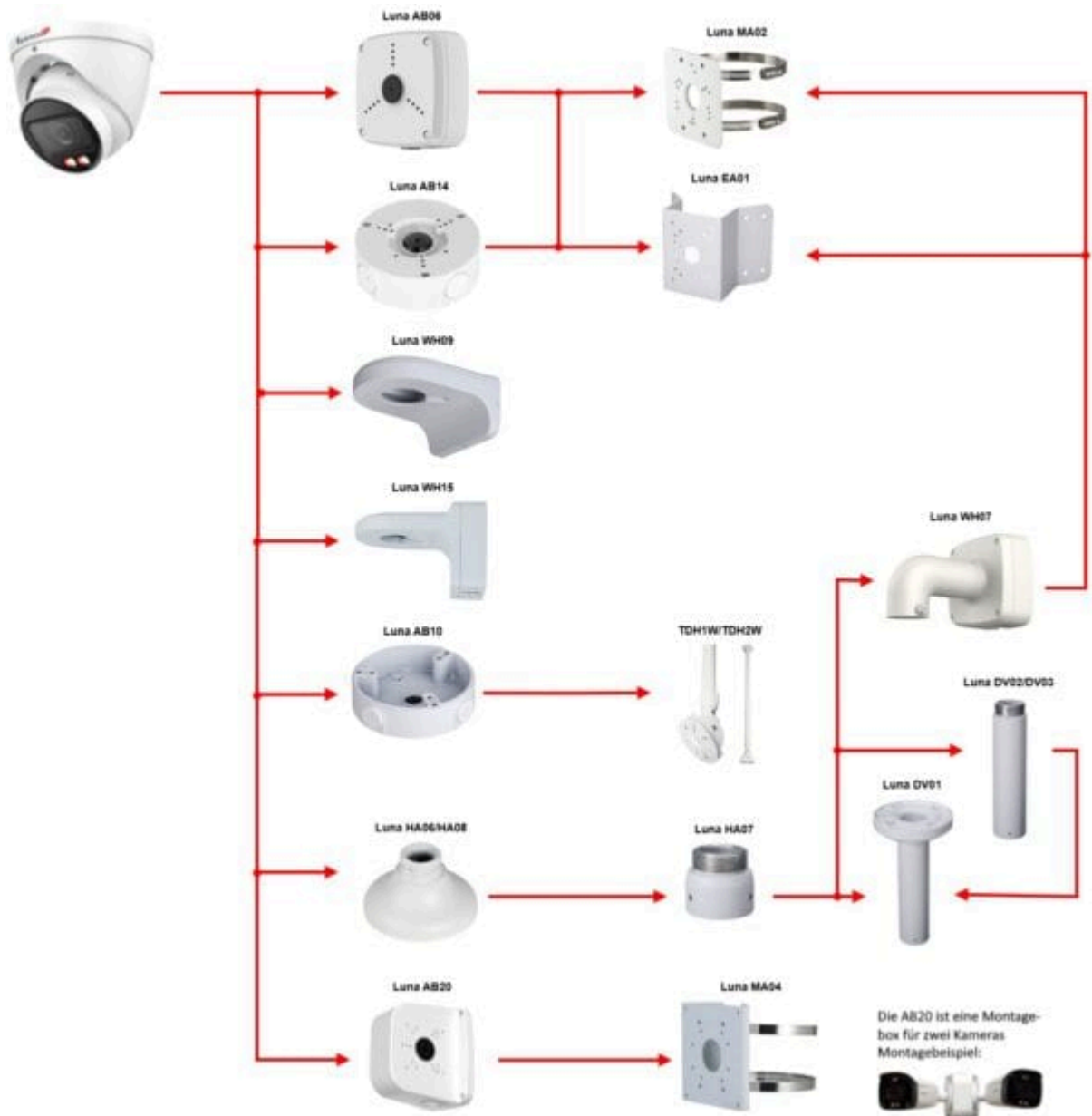
Montageoptionen
