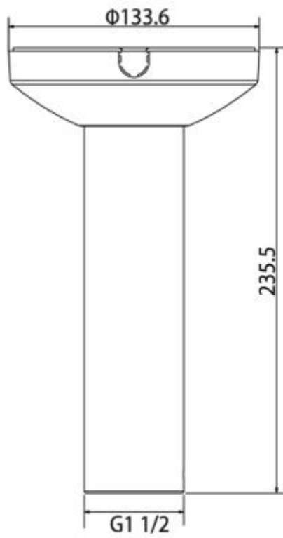
Abmessungen
