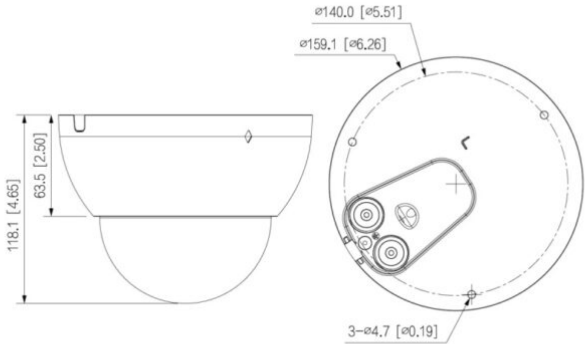
Abmessungen
