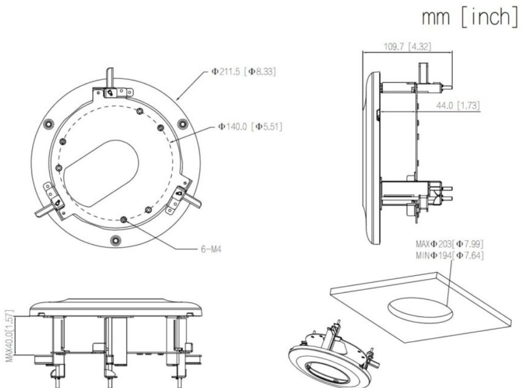
Abmessungen
