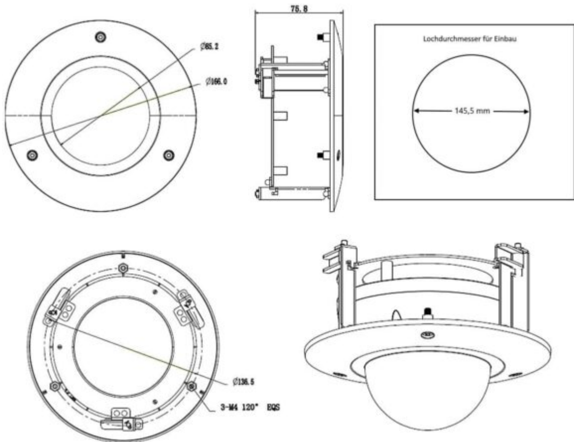
Abmessungen
