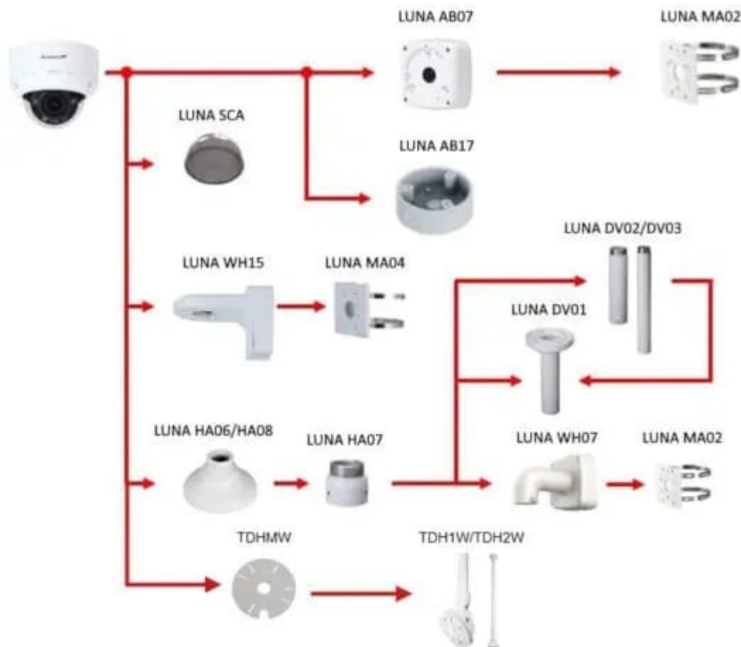
Montageoptionen
