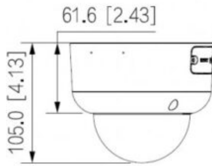
Abmessungen
