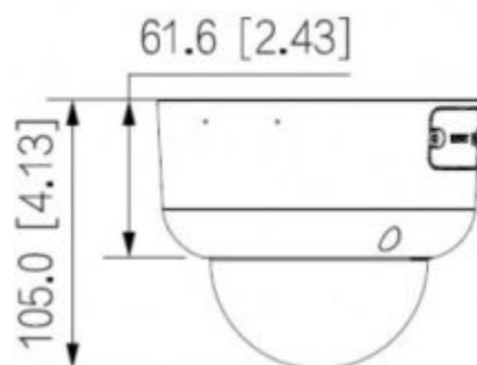
Abmessungen
