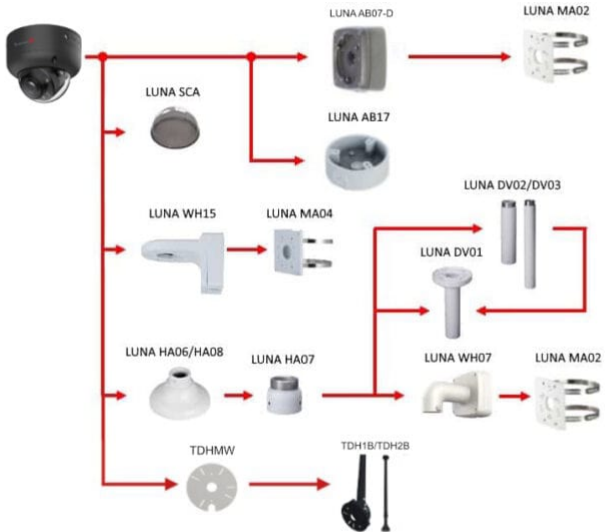
Montageoptionen
