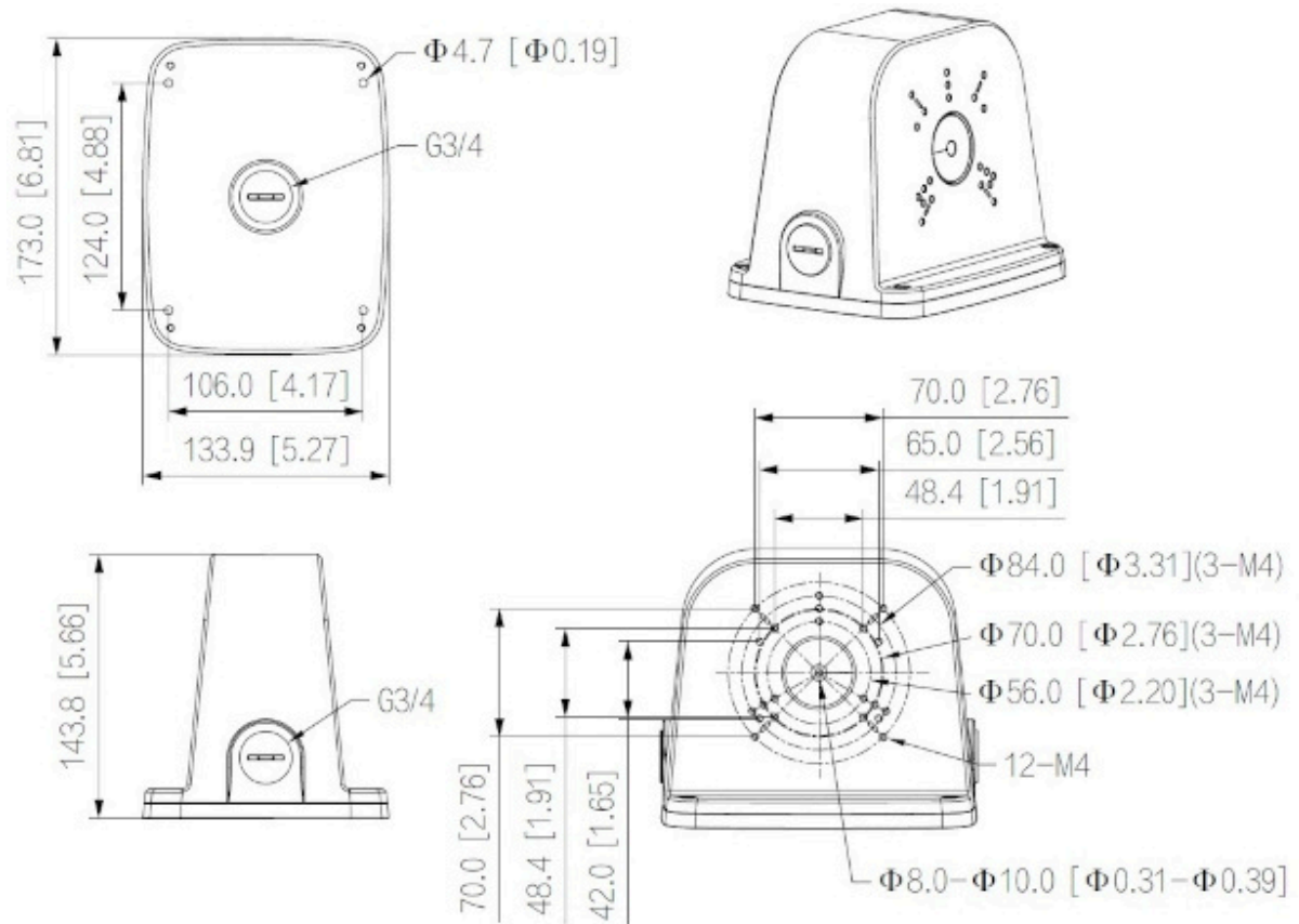
Abmessungen
