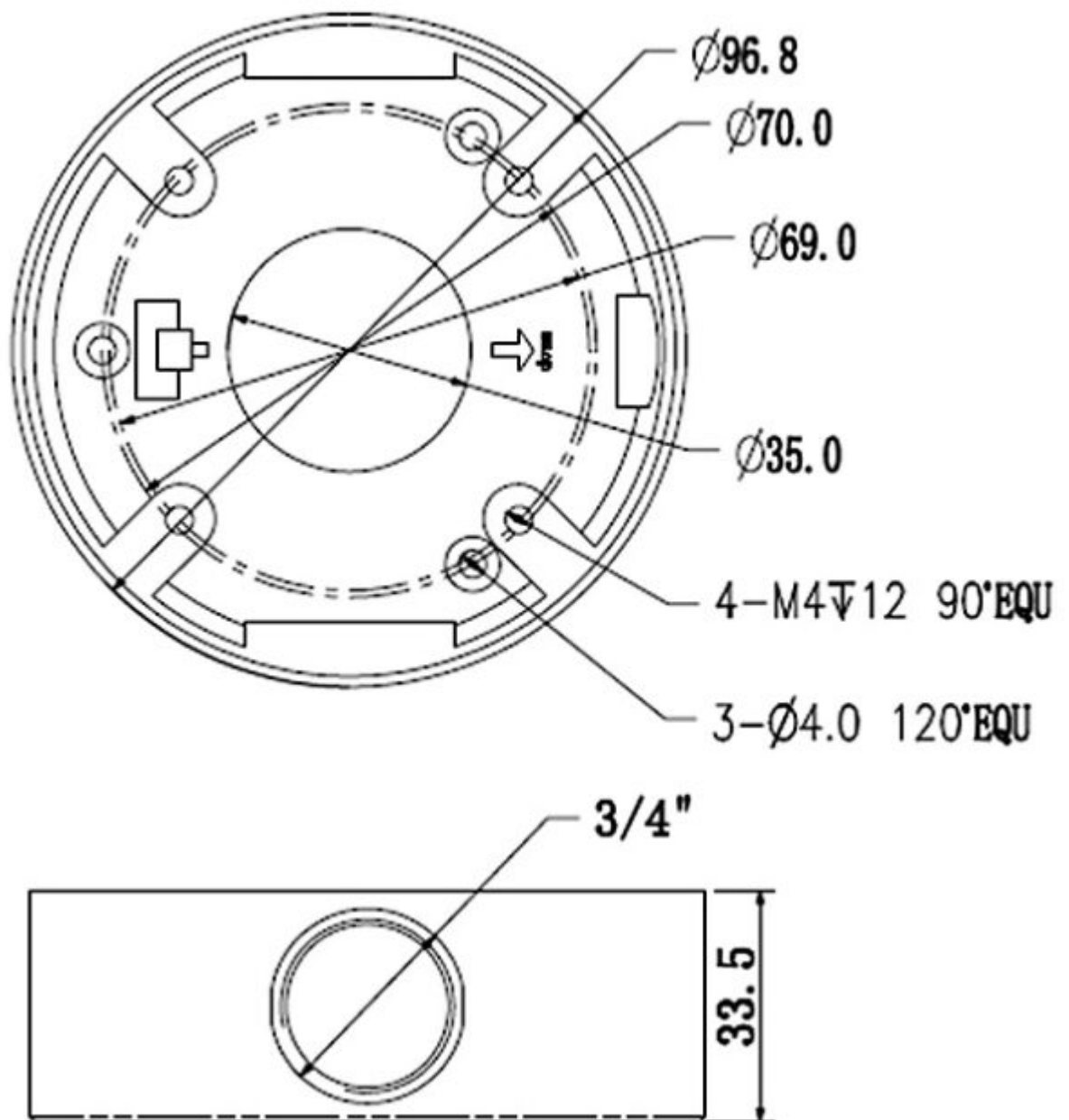
Abmessungen
