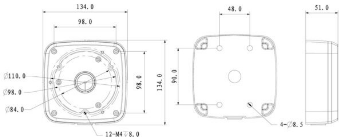
Abmessungen
