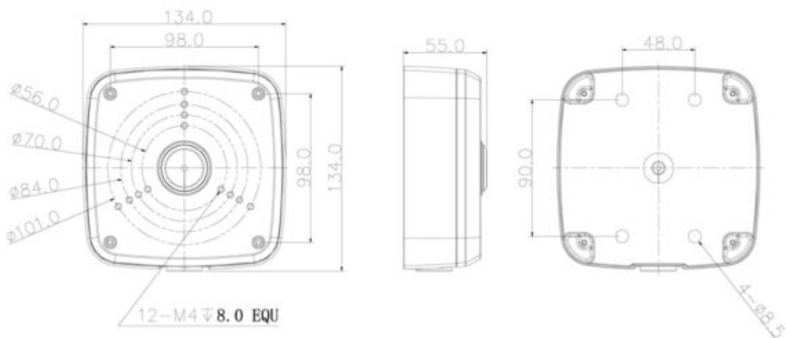
Abmessungen
