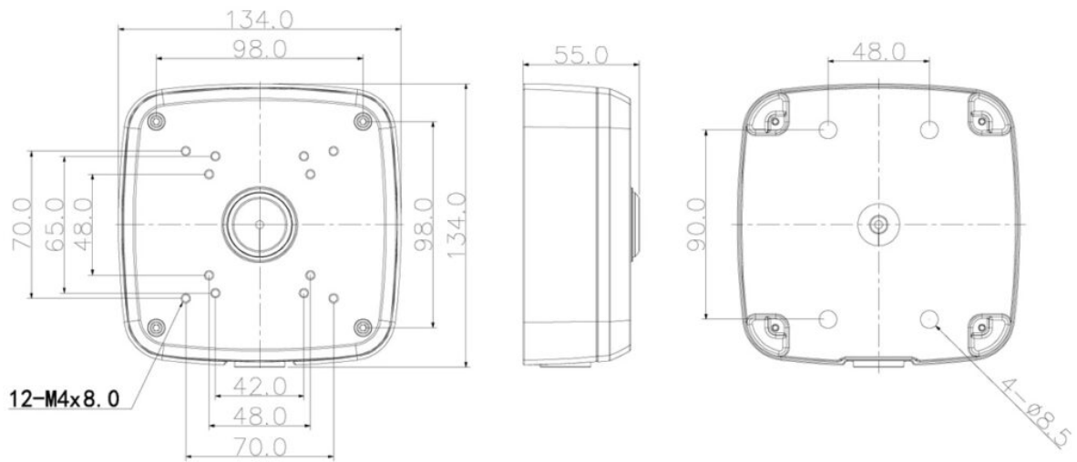
Abmessungen
