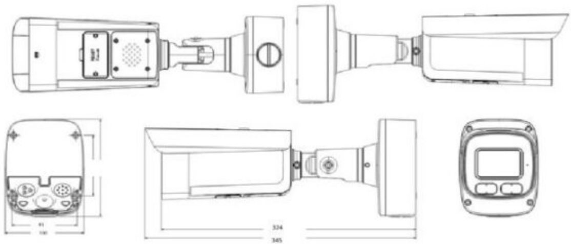
Abmessungen
