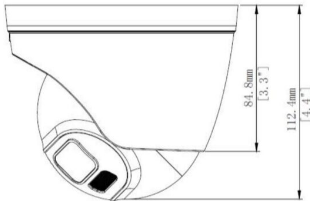
Abmessungen
