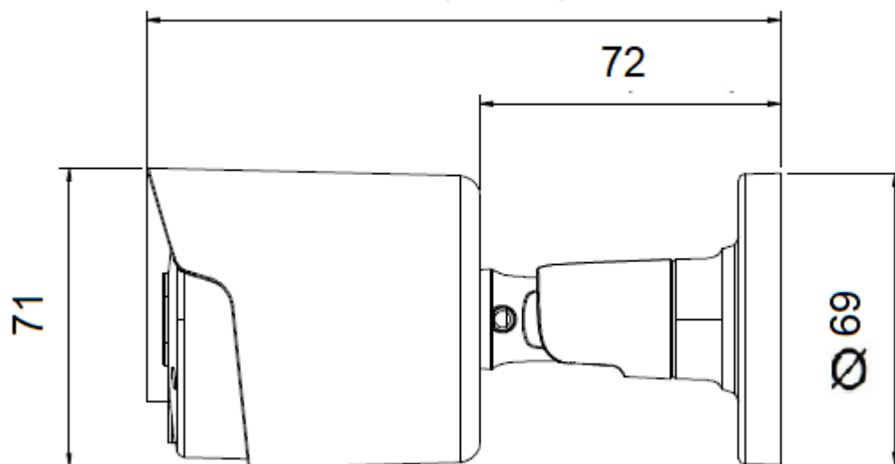
Abmessungen
