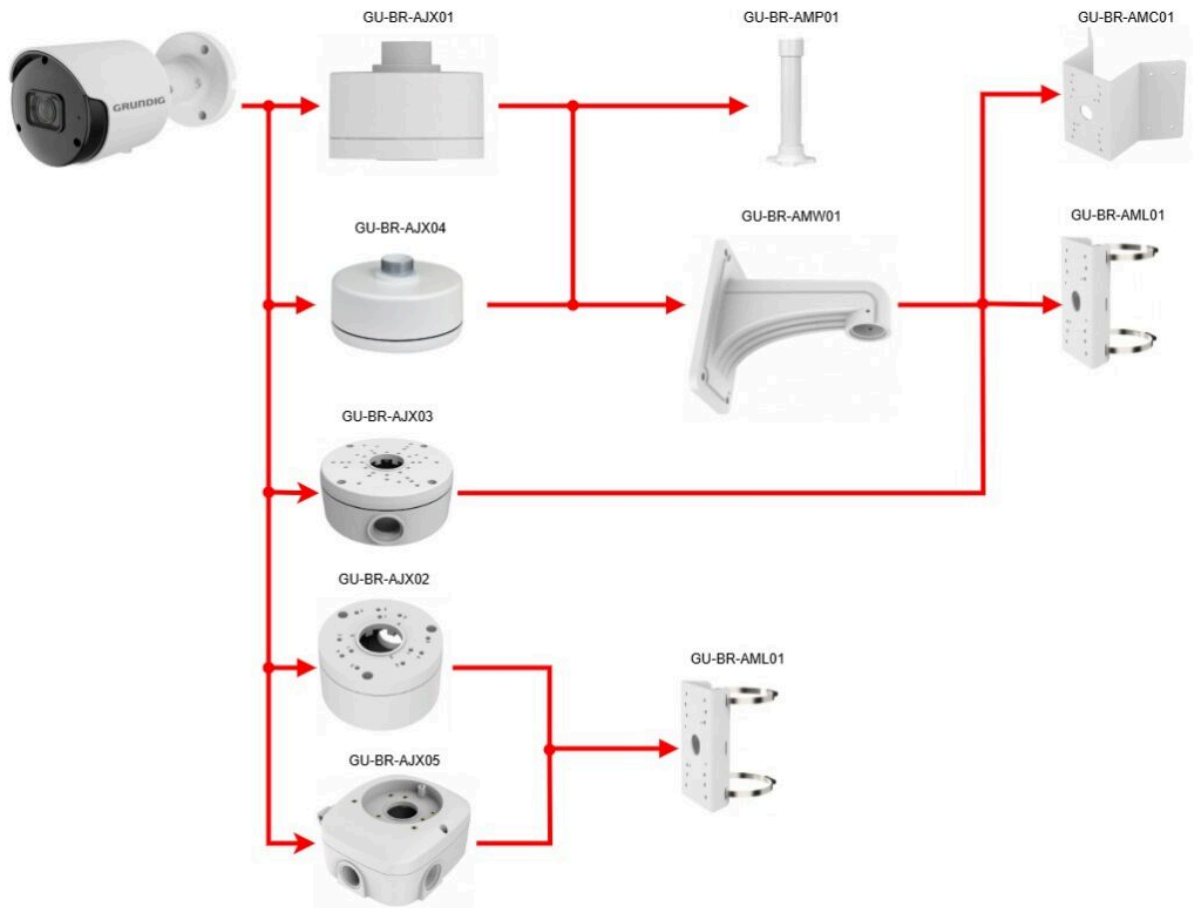
Montageoptionen
