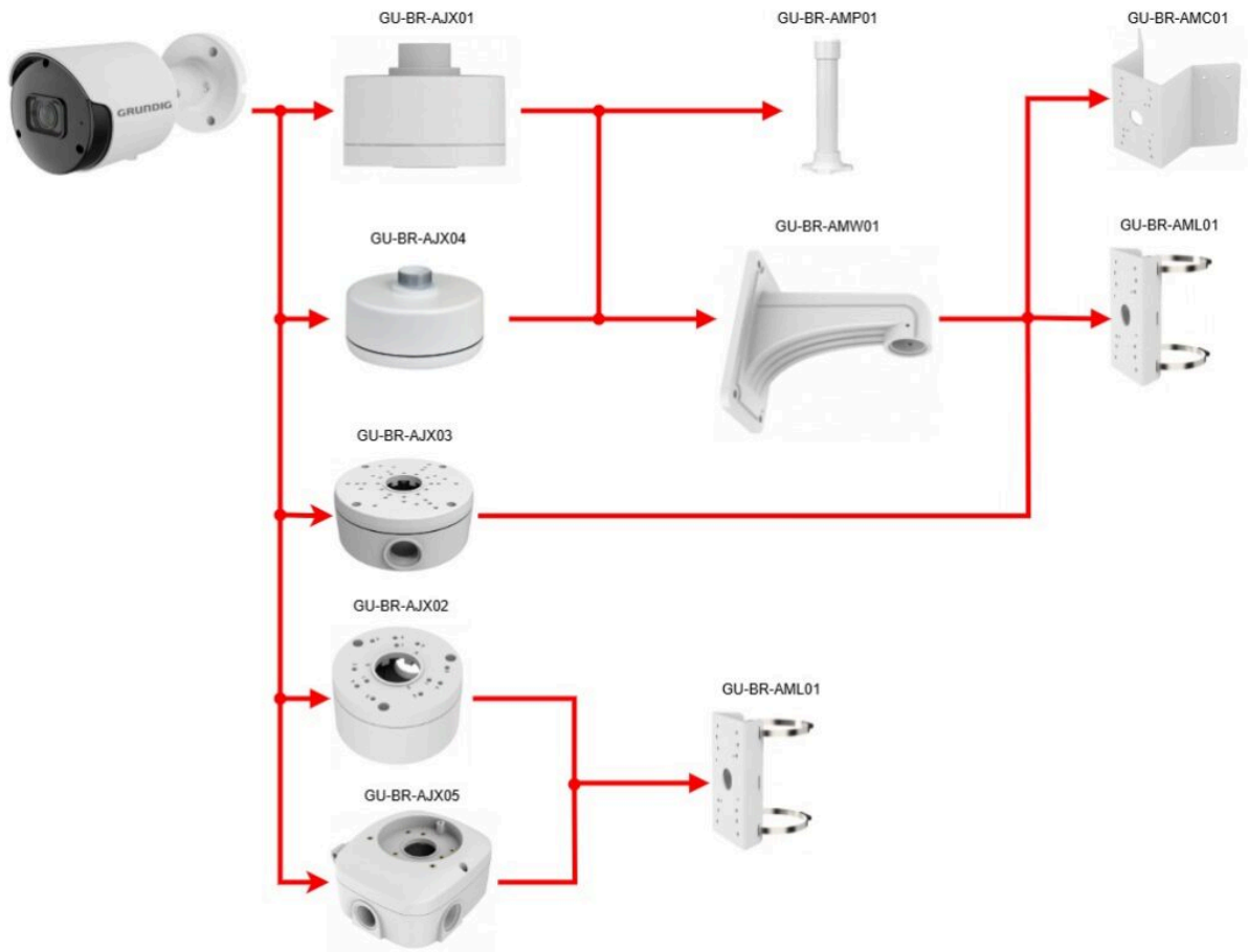
Montageoptionen
