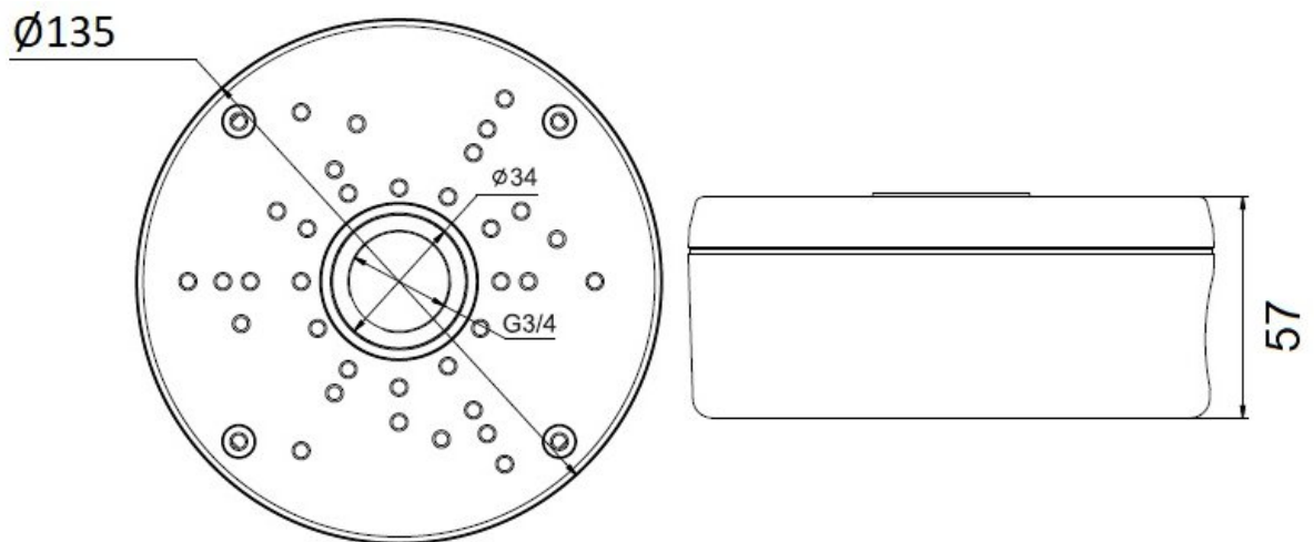
Abmessungen
