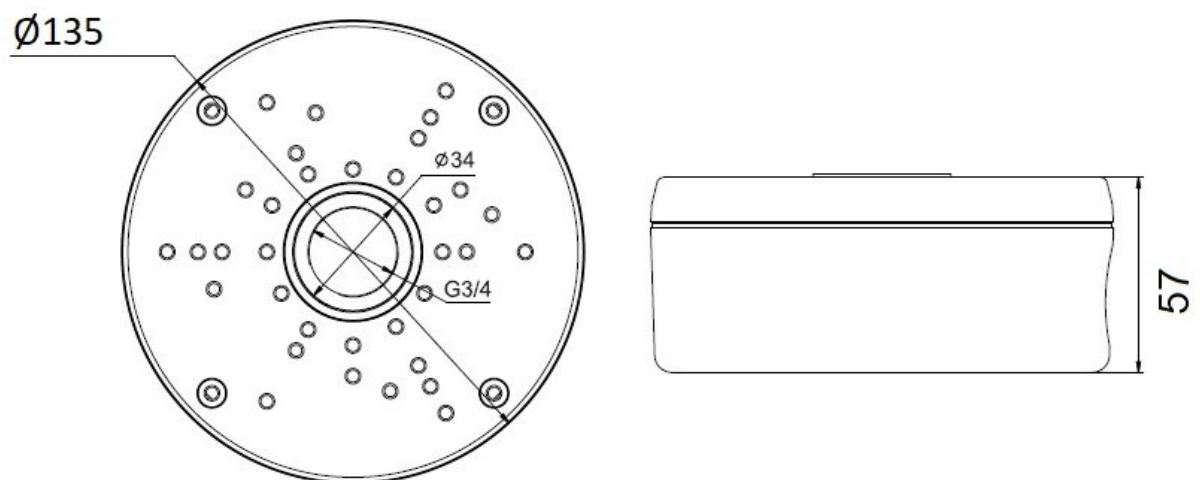
Abmessungen
