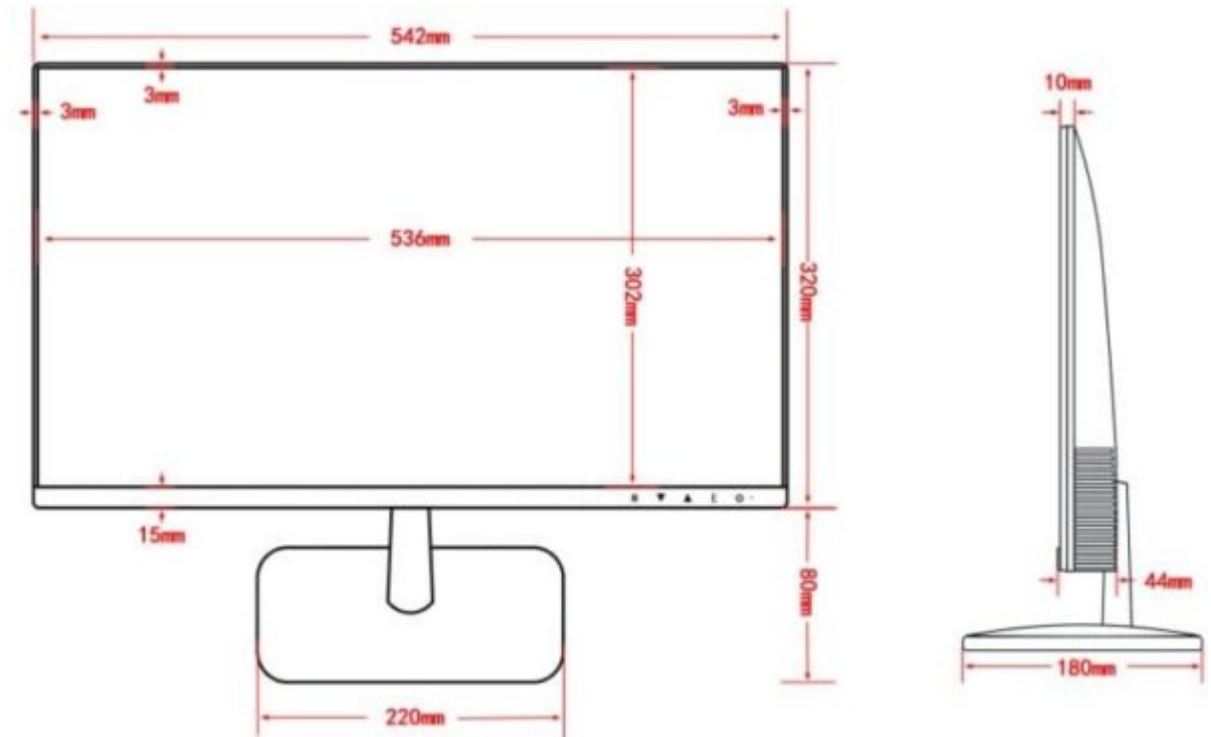
Abmessungen
