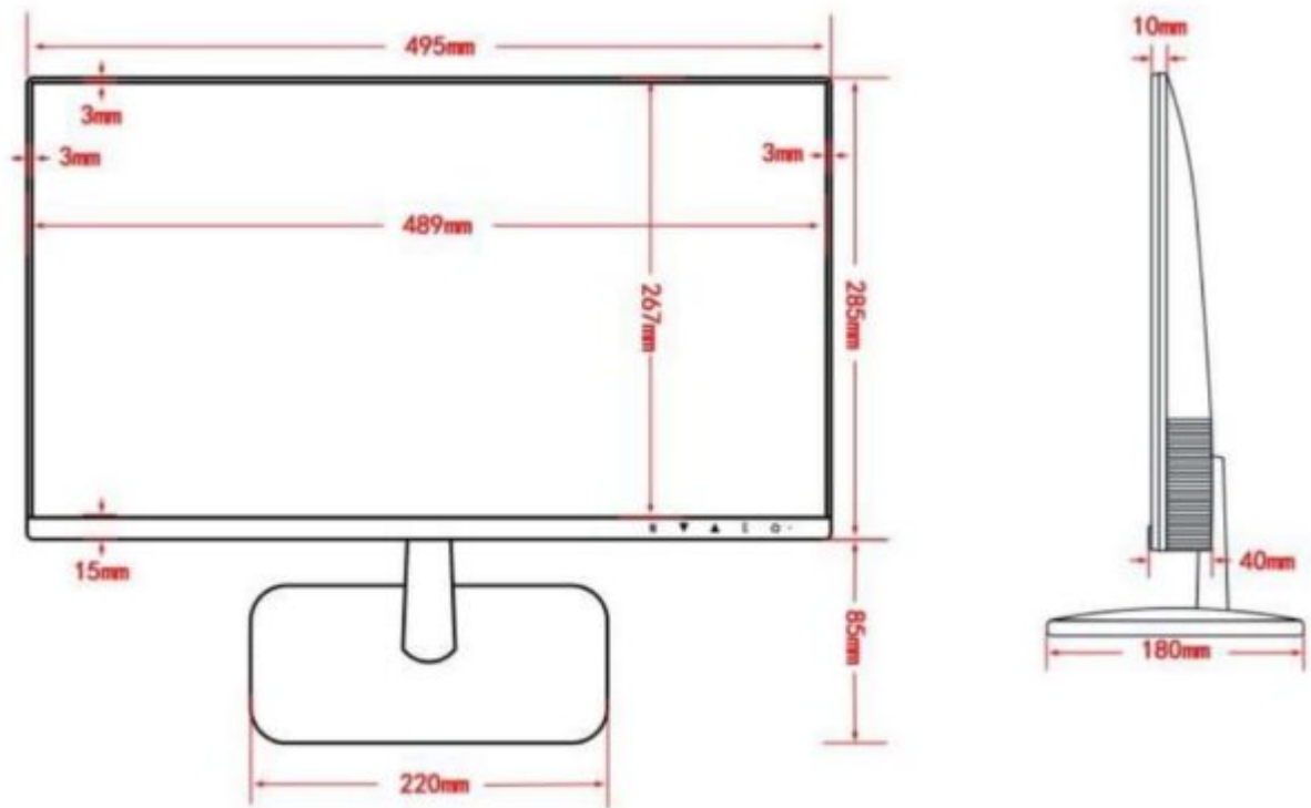
Abmessungen
