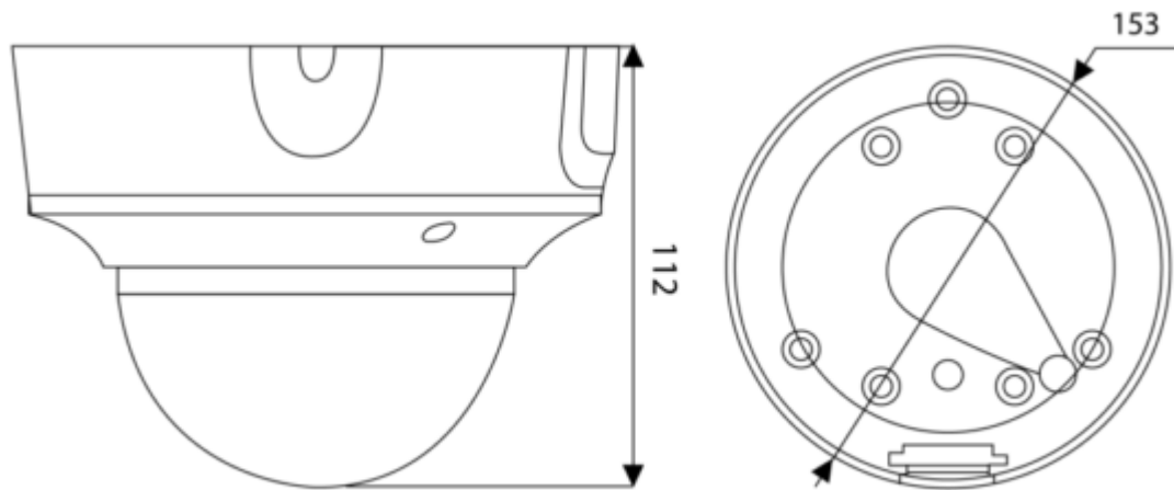
Abmessungen
