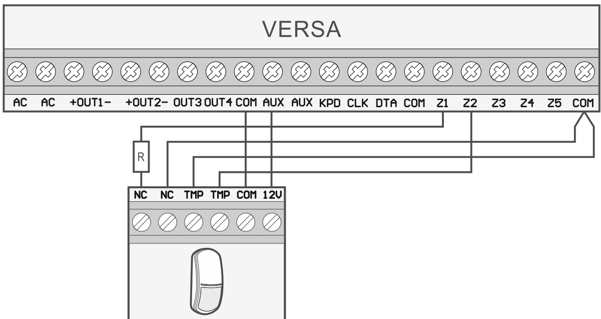
Abb. 23. Beispiel für den Anschluss eines NC-Melders in der Konfiguration EOL.
