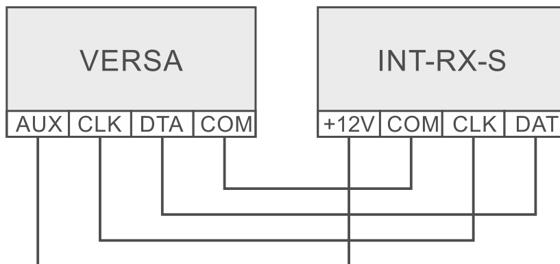
Abb. 8. Anschluss des Erweiterungsmodul INT-RX-S an die Zentrale.
