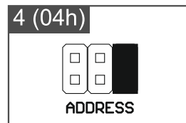
Abb. 7. Adresseinstellung im Modul ETHM-1 Plus (■ - Steckbrücke aufgesetzt; □ - Steckbrücke abgenommen).
