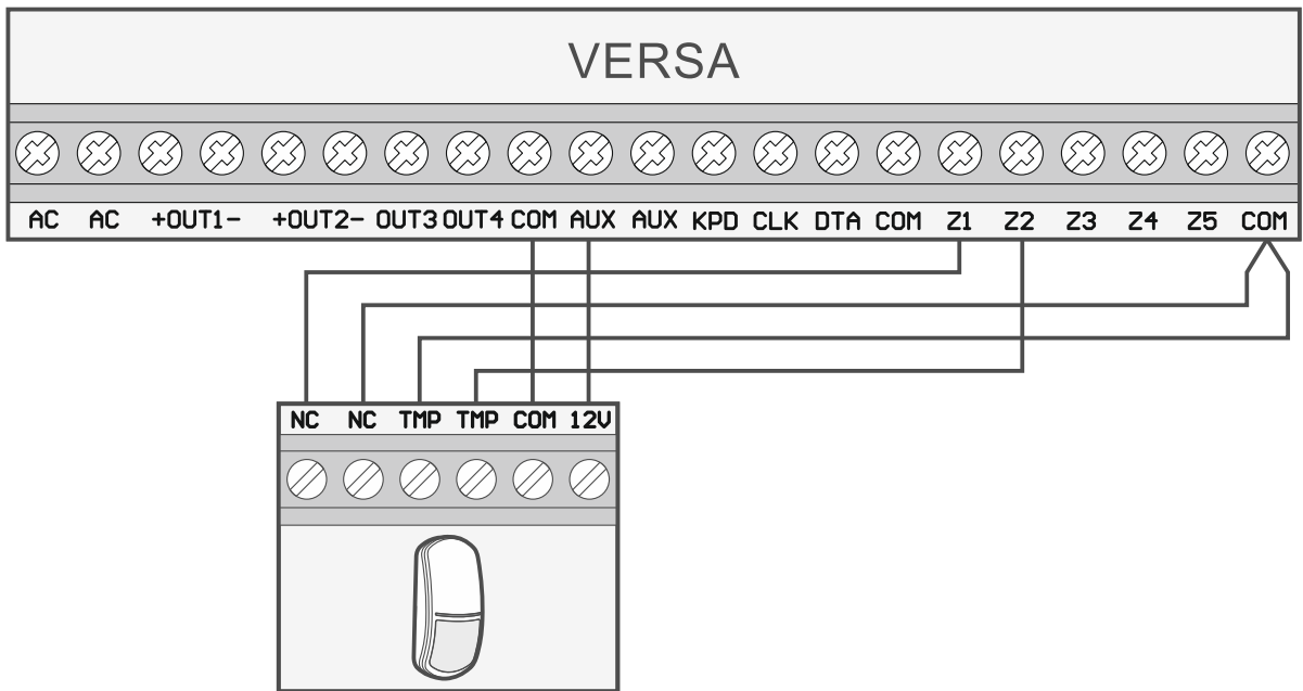
Abb. 22. Beispiel für den Anschluss eines NC-Melders (den NO-Melder schließen Sie identisch an).
