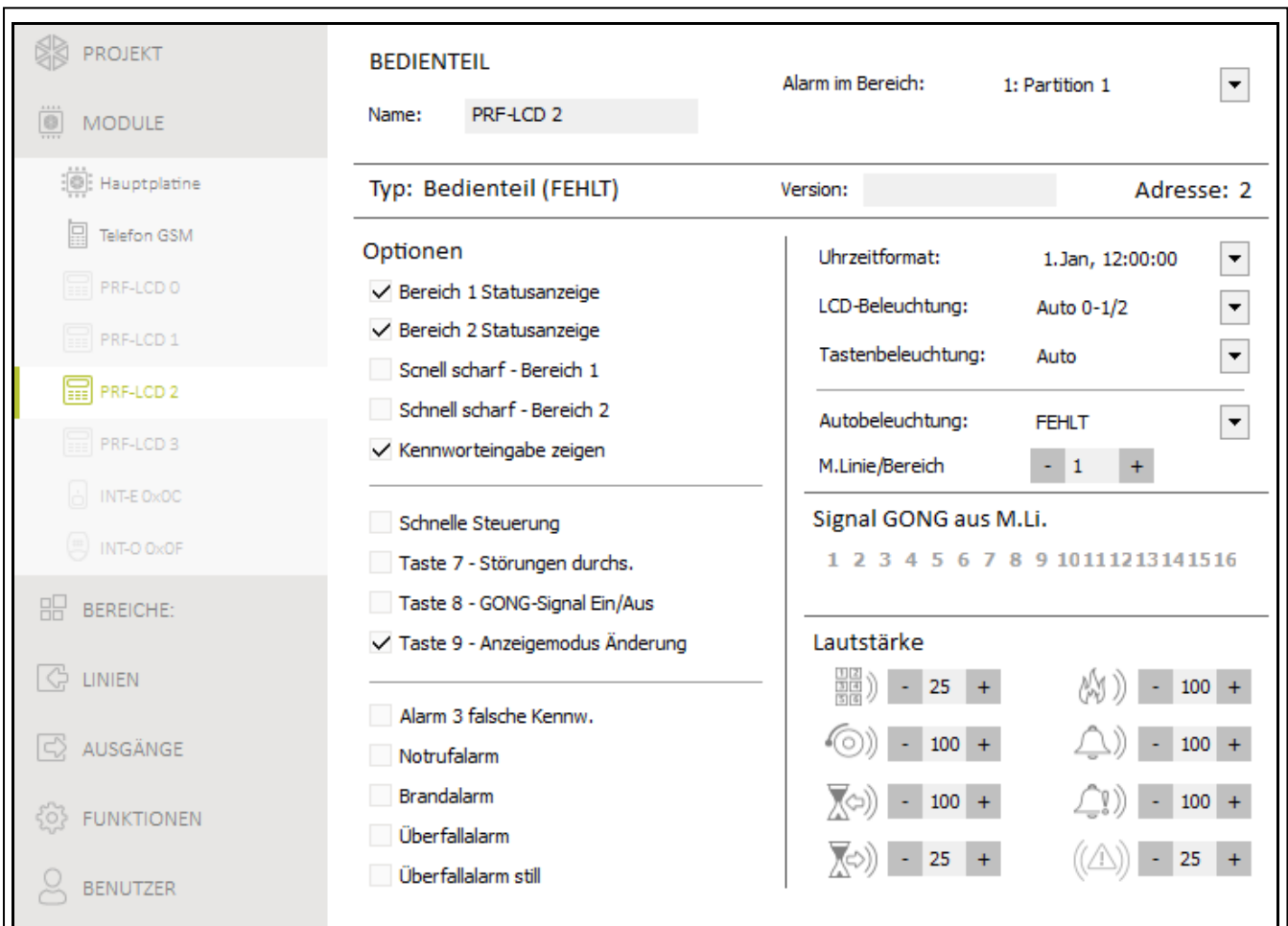
Abb. 10. Registerkarte mit den Einstellungen des verdrahteten Bedienteils.
