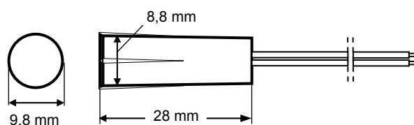
Abb. 2 Reedkontakt im Kunststoffgehäuse (K-2)
