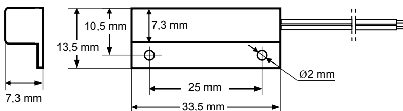
Abb. 1 Reedkontakt im Kunststoffgehäuse (K-1)
