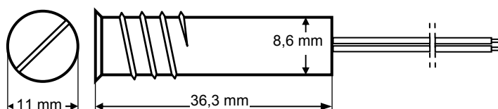
Abb. 3 Reedkontakt im Metallgehäuse (K-3)
