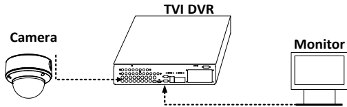
Abbildung 3-1 Anschließen der Geräte
