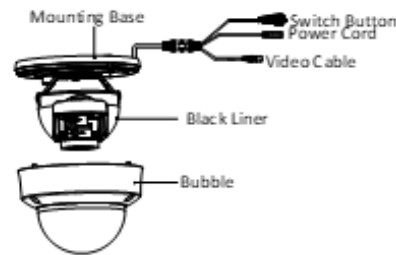
Abbildung 1-1 Kamerakomponenten
