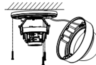
Abbildung 2-3 Kamera befestigen
