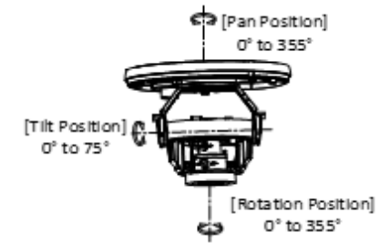
Abbildung 2-4 3-Achsenausrichtung
