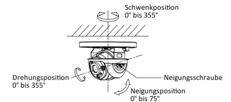
Abbildung 1-5 3-Achsen-Einstellung
