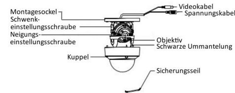
Abbildung 1-1 Kamerakomponenten
