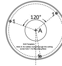
Abbildung 1-2 Die Bohrschablone
