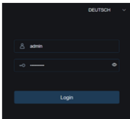
Abbildung 4-1 Login Oberfläche
