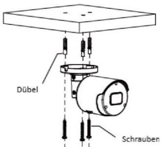
Abbildung 2-3 Kamera an Wand/Decke befestigen
