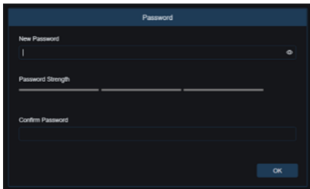
Abbildung 3-3 Aktivierungsoberfläche (Web)
