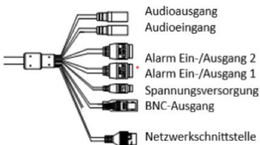
Abbildung 1-2 Beschreibung Kabelbaum
