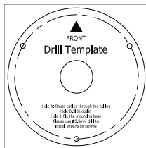
Abbildung 2-4 Bohrschablone
