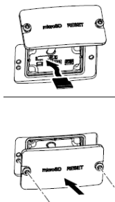
Abbildung 2-2 Einsetzen der Speicherkarte
