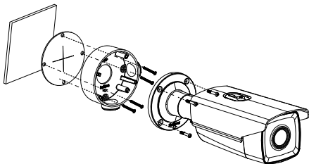
Abbildung 2-5 Anschlussbox befestigen
