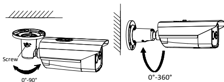
Abbildung 2-6 Kamerajustage
