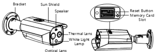
Abbildung 1-1 Beschreibung der Kamera
