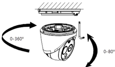
Abbildung 2-4 Kamera ausrichten
