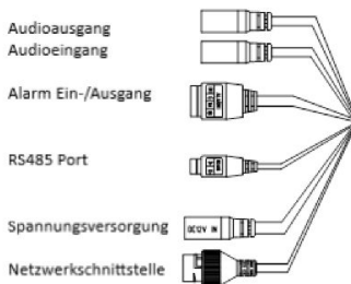
Abbildung 1-2 Beschreibung Kabelbaum
