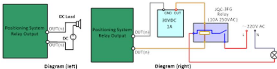
Abbildung 1-3 Beschreibung Alarmausgang
