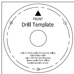
Abbildung 2-1 Bohrschablone
