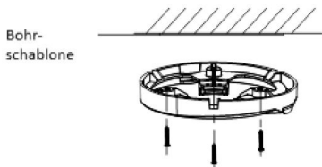
Abbildung 2-3 Sockel montieren
