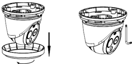
Abbildung 2-2 Ring entfernen
