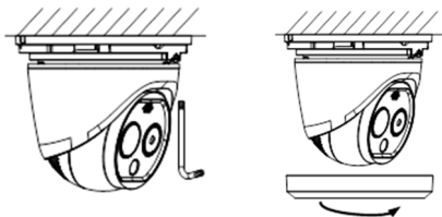
Abbildung 2-5 Montage auf Sockel
