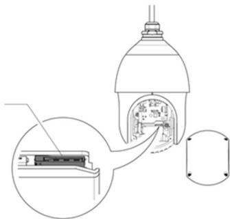
Abbildung 2-2 Installation der SD-Karte
