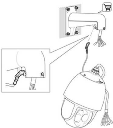
Abbildung 2-5 Sicherungsseil anbringen
