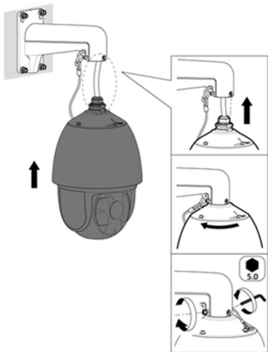
Abbildung 2-6 Kamera befestigen
